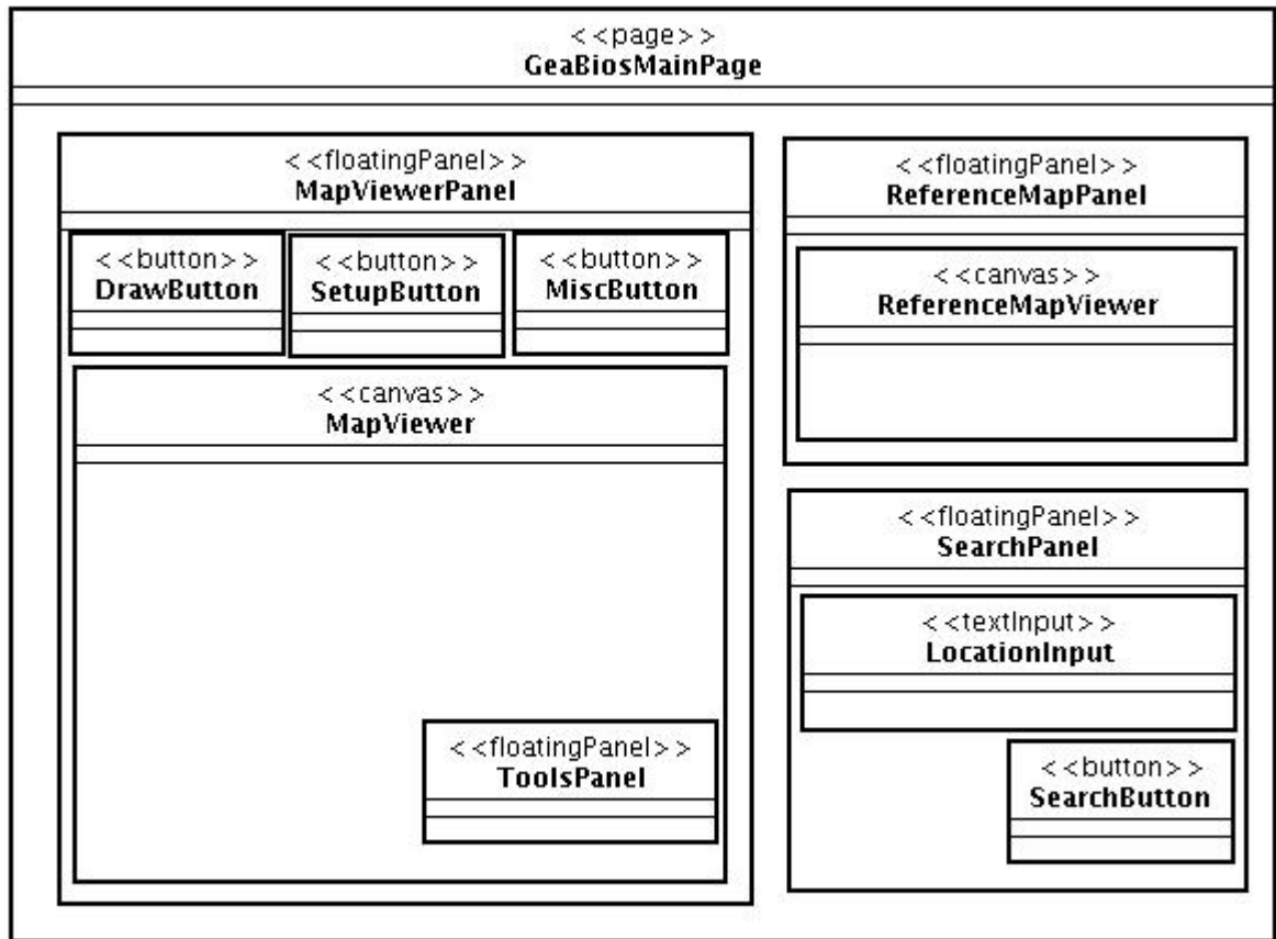
Figura 28 – UWE-R para GeaBios: modelo de apresentação
