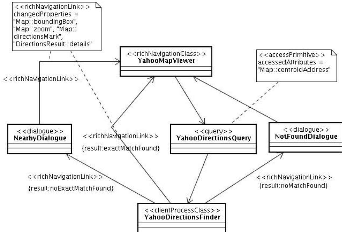
Figura 29 – UWE-R para Yahoo! Maps: modelo de navegação
