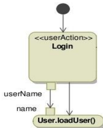
Figura 11 – UWE: Excerto de diagrama de atividade (KROIB; KOCH , 2008)
