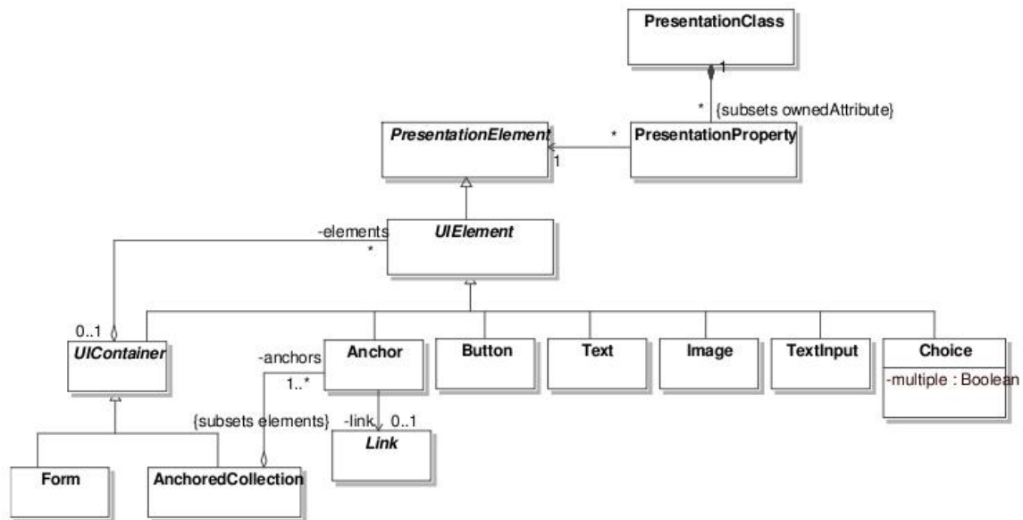
Figura 9 – UWE: elementos de interface gráfica (KROIB; KOCH , 2008)
