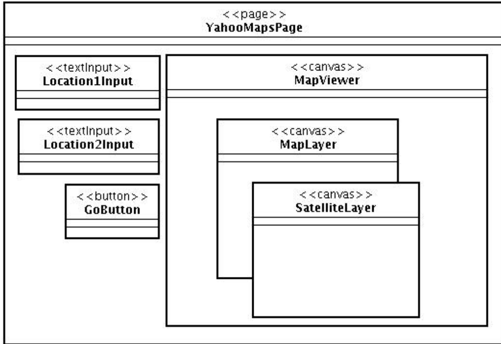
Figura 32 – UWE-R para Yahoo! Maps: modelo de apresentação
