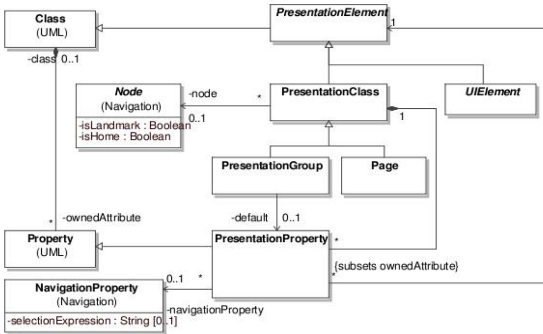
Figura 8 – UWE: pacote de apresentação (KROIB; KOCH , 2008)
