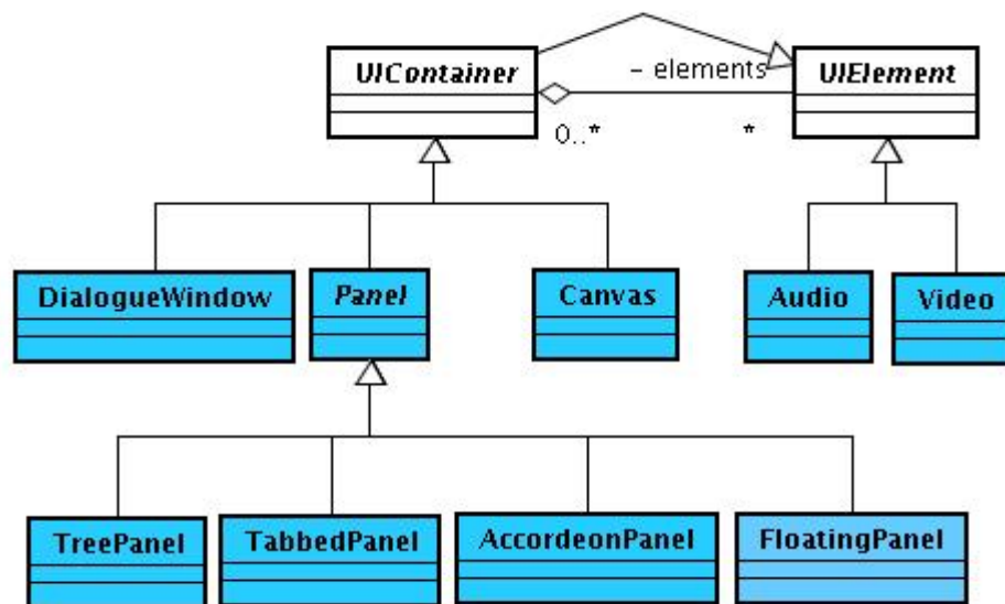
Figura 15 – UWE-R: novas metaclassas de apresentação
