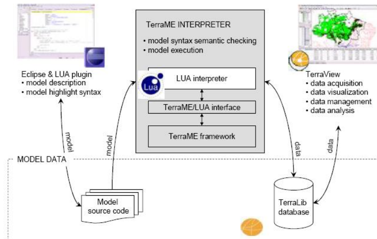
Figura 9 - Módulos do TerraME. Fonte: Carneiro (2006).
