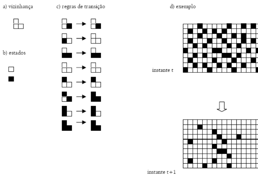
Figura 5 - Estrutura de um autômato celular (AC).
