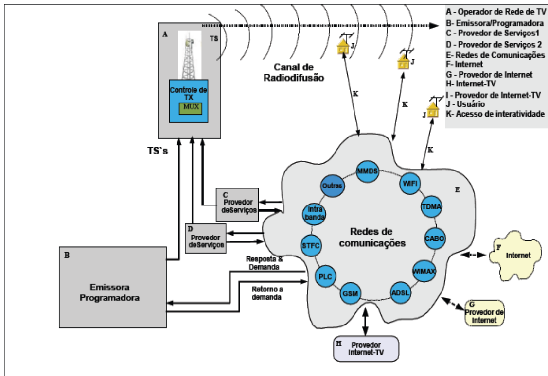
Figura 13 – Redes de Comunicação para constituir o Canal de Retorno (CPQD, 2006)
