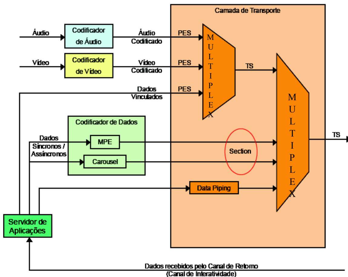
Figura 09 – Transmissão de Dados (CPQD, 2006).
