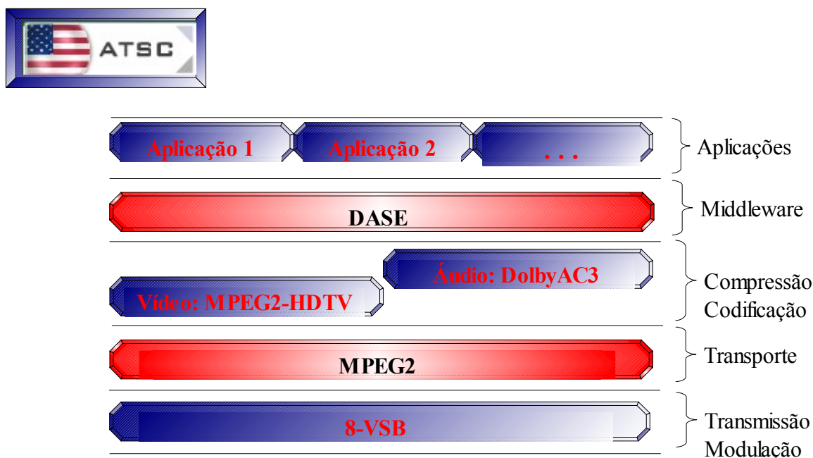
Figura 01 – Camadas do Padrão de TV Digital ATSC (FERNANDES, 2004).
