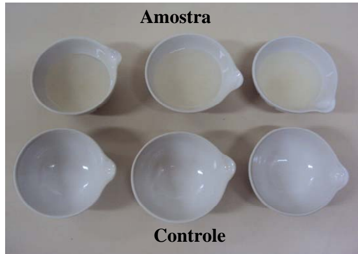
Figura 2.20 Cadinhos para o controle dos sólidos totais
