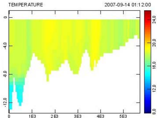
Figura 21 - Temperatura da água com a ocorrência de ventos no reservatório na simulação Primavera-V.
