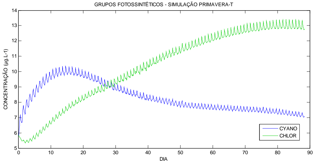
Figura 28 - Variação dos grupos fotossintéticos (cianobactérias e clorofíceas) no reservatório do Lobo na simulação Primavera-T.
