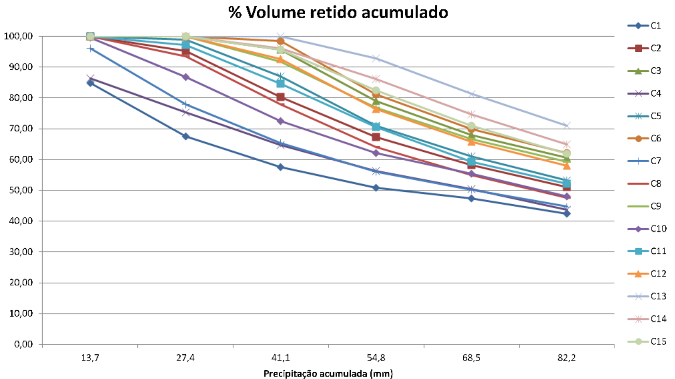
Gráfico 5. Desempenho da capacidade de retenção hídrica (%) das colunas no Pré-ensaio.
