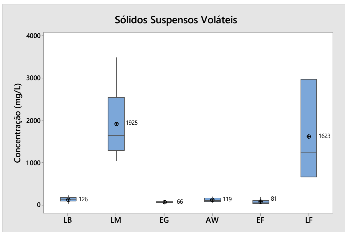
Figura 25 - Representação gráfica (box-plot) da distribuição dos valores sólidos suspensos voláteis.
