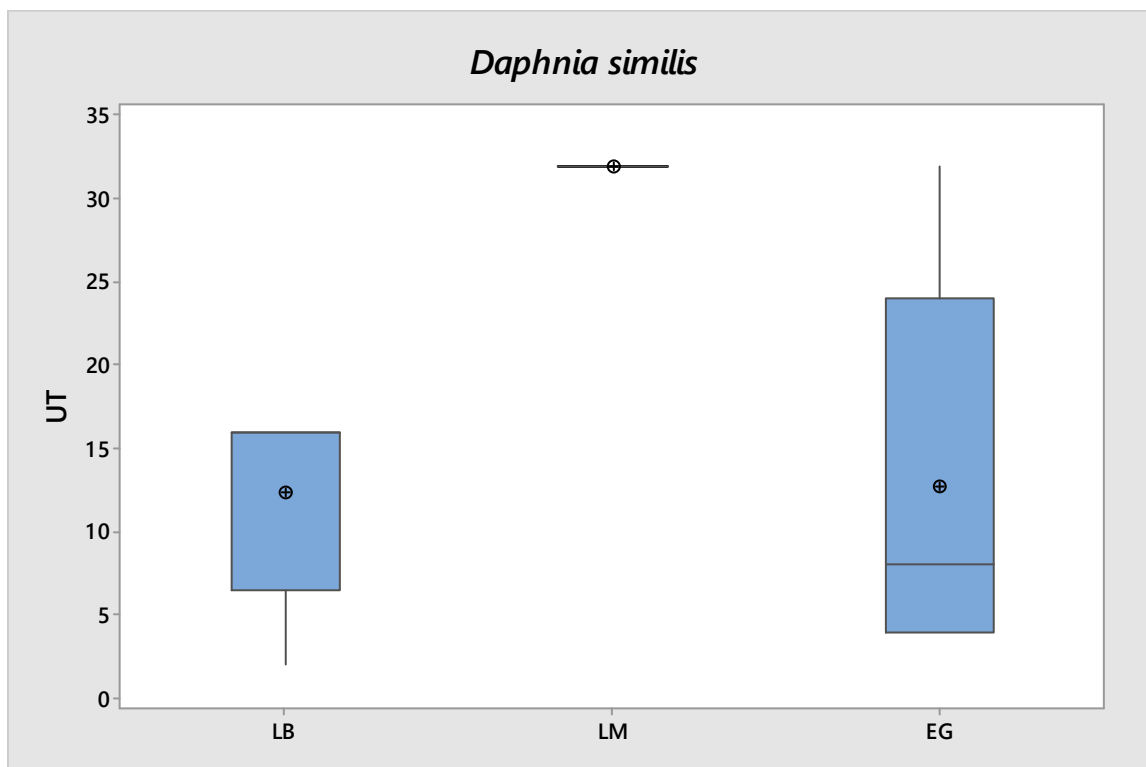
Figura 30 - Representação gráfica (boxplot) do valores de UT para Daphnia similis .
