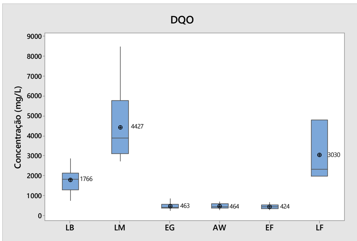
Figura 20 –Representação gráfica (box-plot) da distribuição dos valores de DQO.
