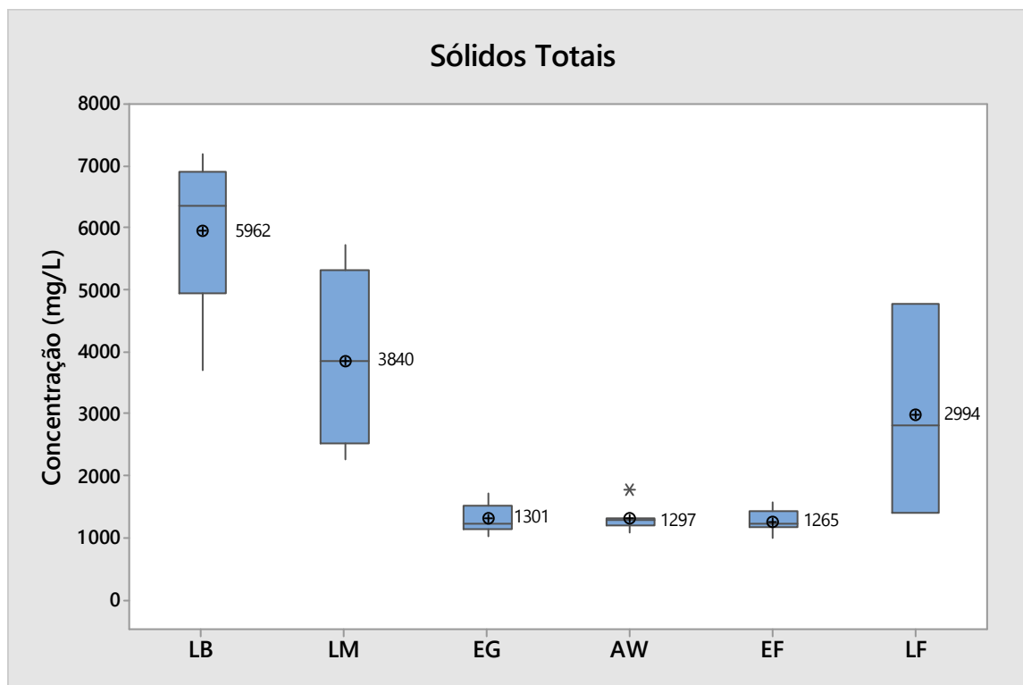
Figura 23- Representação gráfica (box-plot) da distribuição dos valores de sólidos totais.
