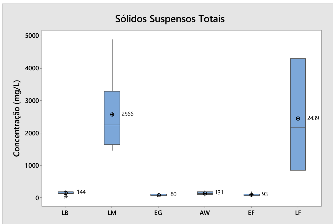
Figura 24 - Representação gráfica (box-plot) da distribuição dos valores de sólidos suspensos totais
