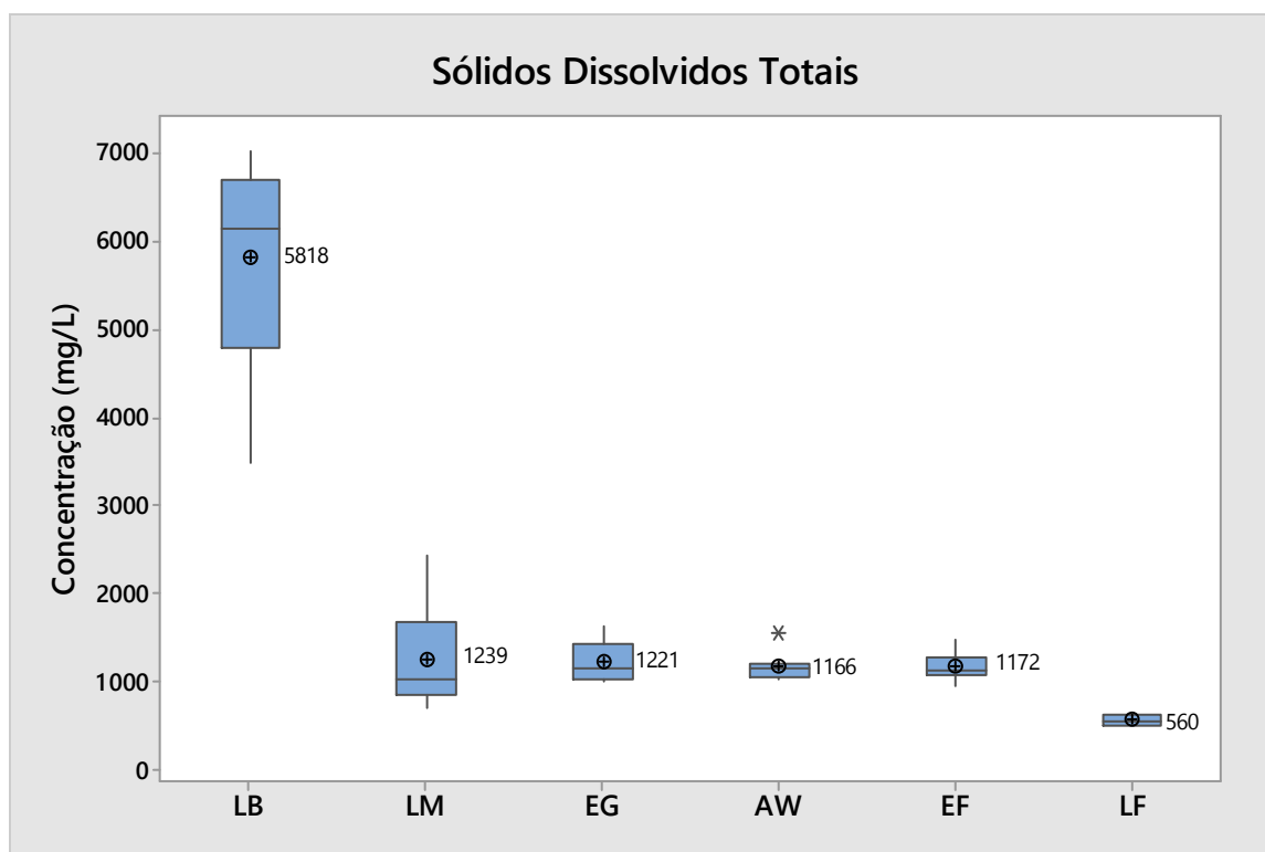
Figura 26 - Representação gráfica (box-plot) da distribuição dos valores de sólidos dissolvidos totais.
