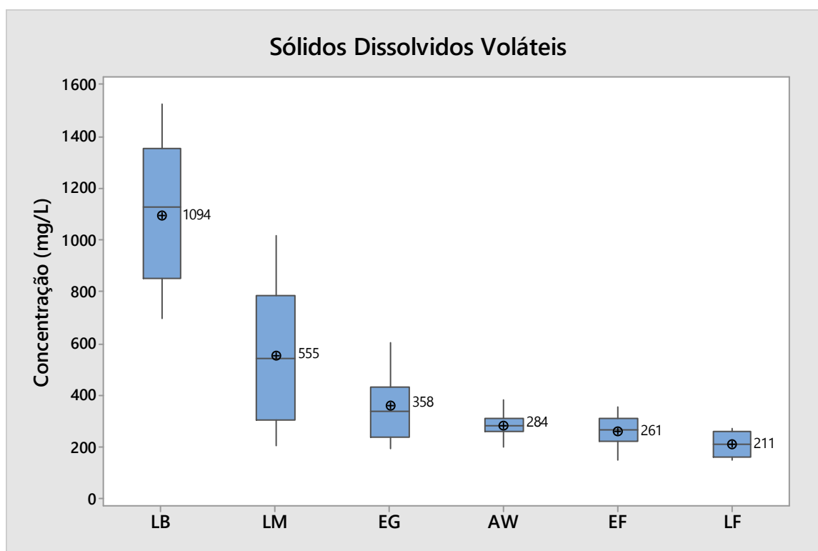
Figura 27 - Representação gráfica (box-plot) da distribuição dos valores de sólidos dissolvidos voláteis.
