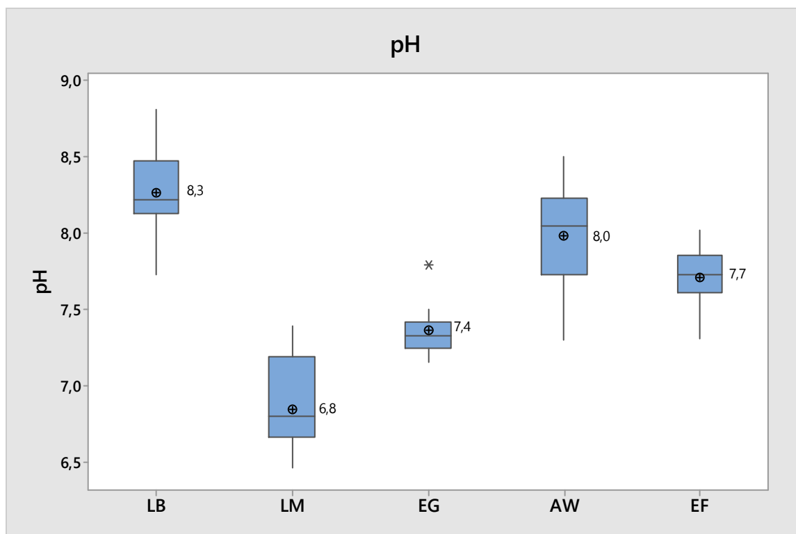
Figura 18 - Representação gráfica (boxplot) dos valores de pH.
