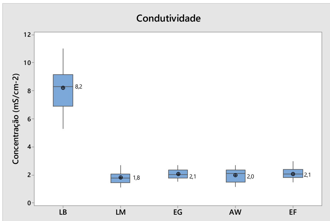
Figura 19 - Representação gráfica (boxplot) dos valores de condutividade.
