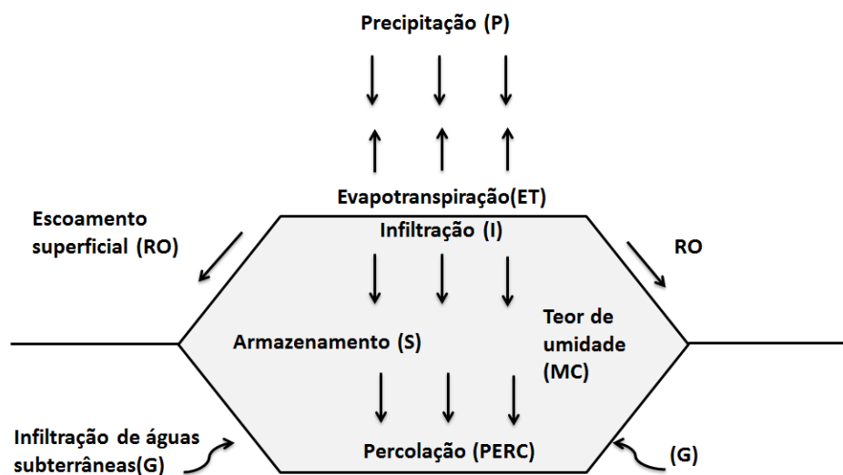
Figura 1 - Balanço hídrico da formação de lixiviado.
