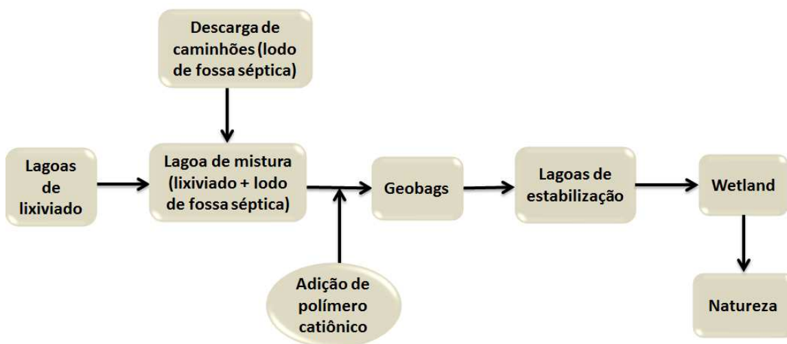
Figura 9 - Esquema da estação de tratamento de lixiviado e lodo de fossa séptica do aterro.
