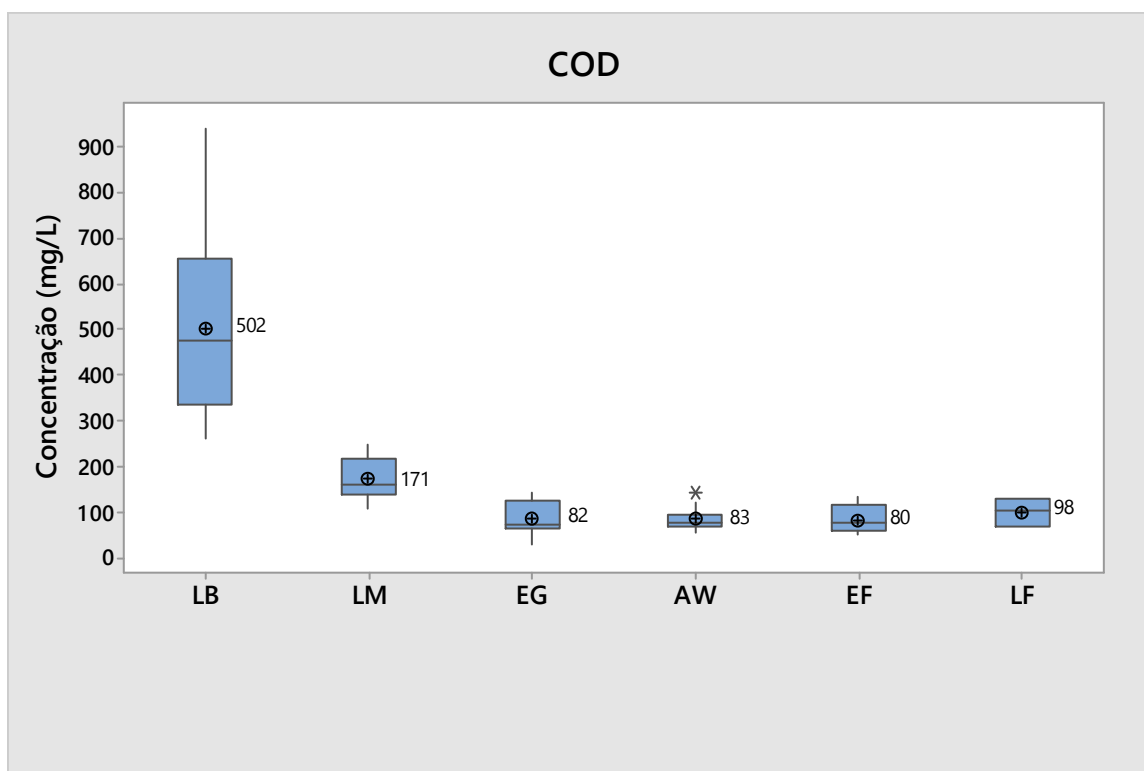
Figura 21- Representação gráfica (box-plot) da distribuição dos valores de COD.
