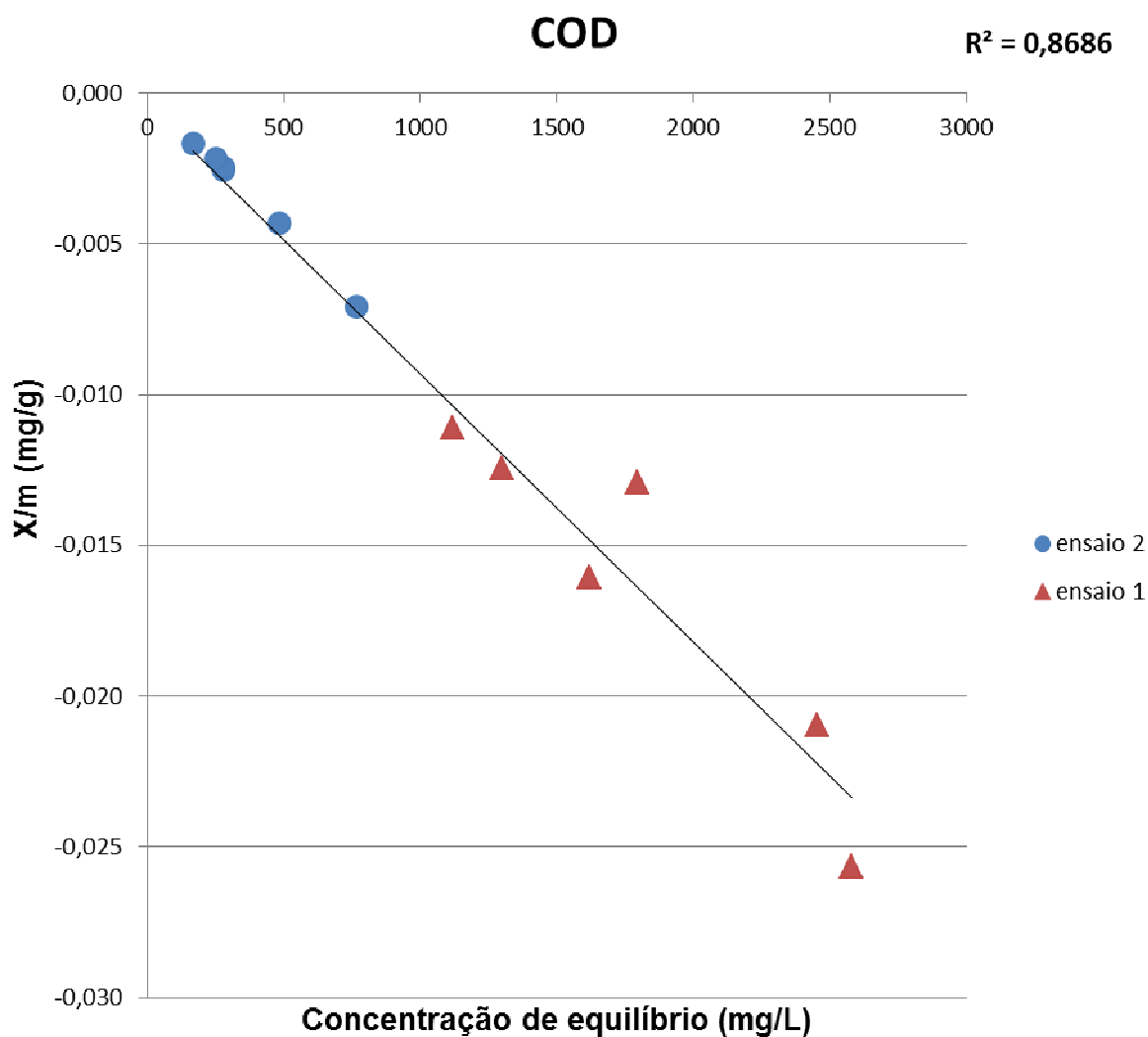
Figura 28 - Sorção de COD nos ensaios 1 e 2.
