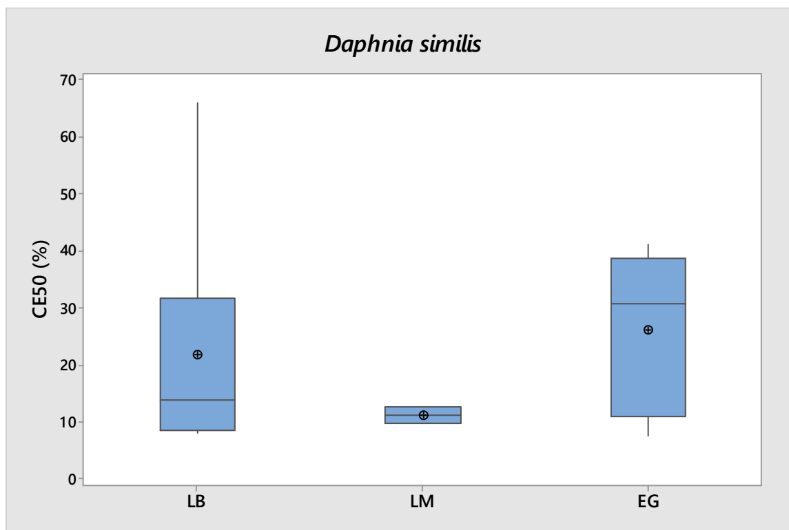
Figura 31 - Representação gráfica (boxplot) dos valores de CL50(%) para Daphnia similis .
