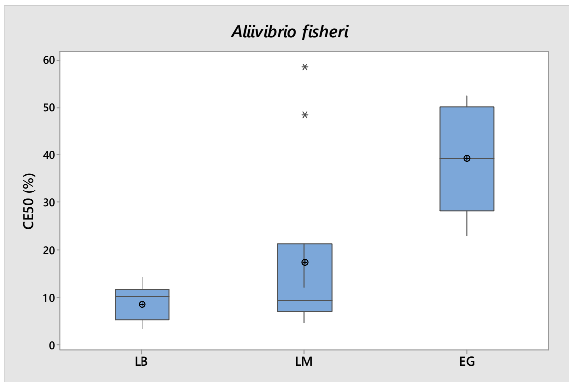
Figura 33 - Representação gráfica (boxplot) dos valores de CL50(%) para Aliivibrio fischeri .
