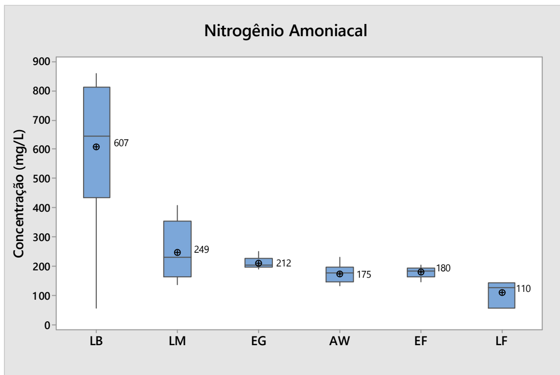
Figura 22 - Representação gráfica (box-plot) da distribuição dos valores de nitrogênio amoniacal.
