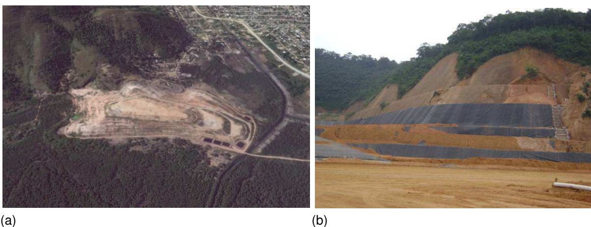
Figura 7 – Aterro controlado de Itaoca
