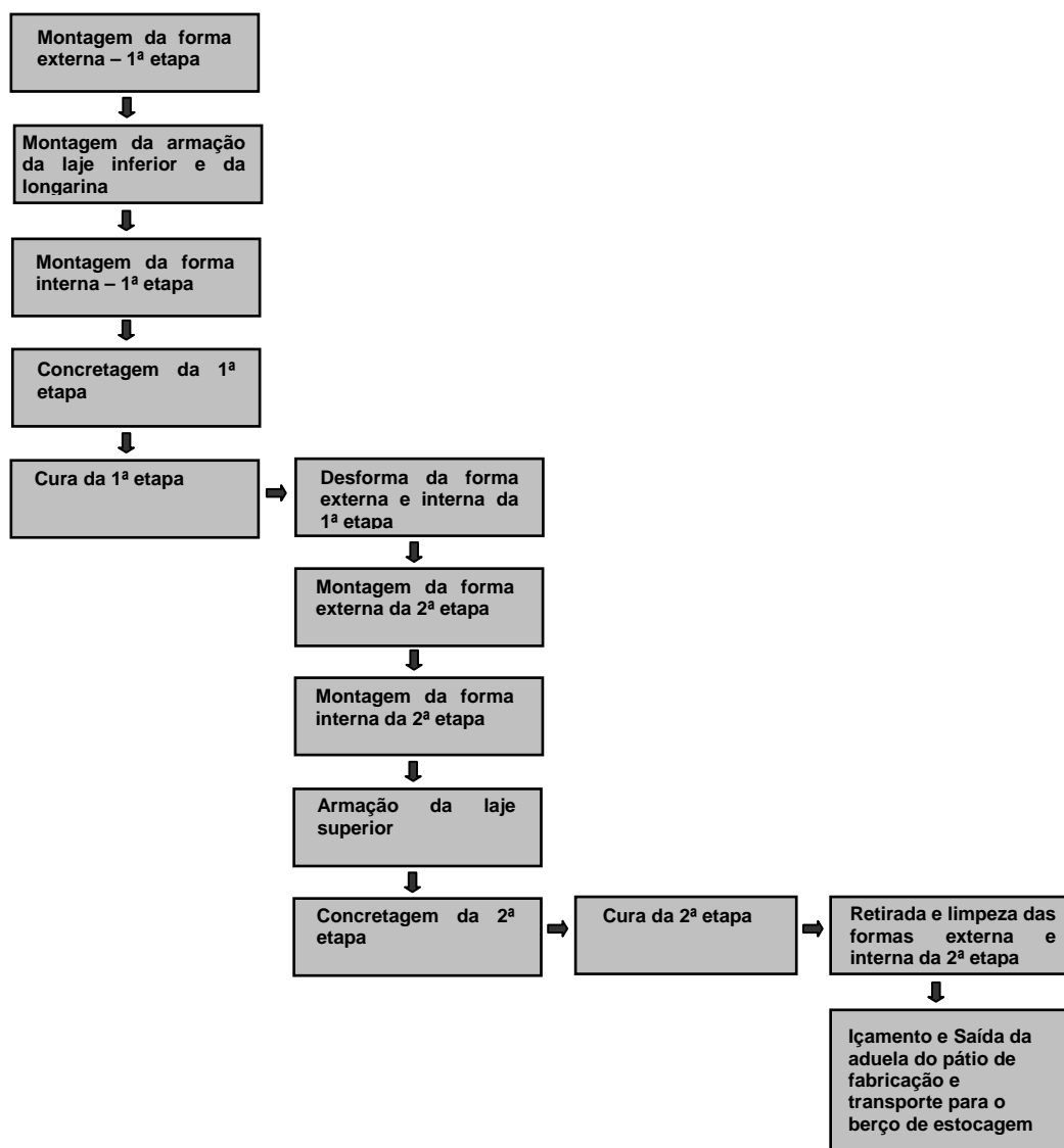
Figura 5.51 - Processo de fabricação com concretagem em duas etapas.
