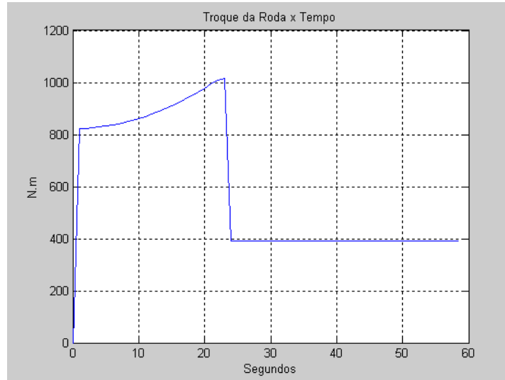
Figura 39 - Torque na roda, em N.m, versus tempo referente ao item 3.7.4
