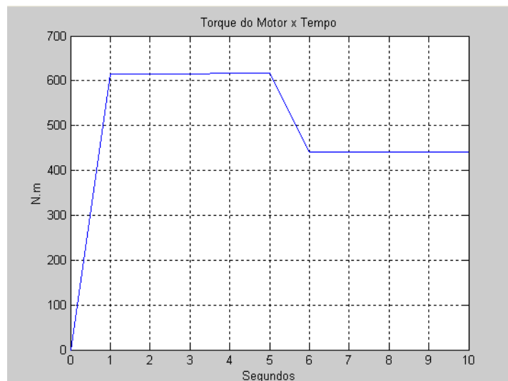
Figura 36 - Torque no motor, em N.m, versus tempo referente ao item 3.7.3
