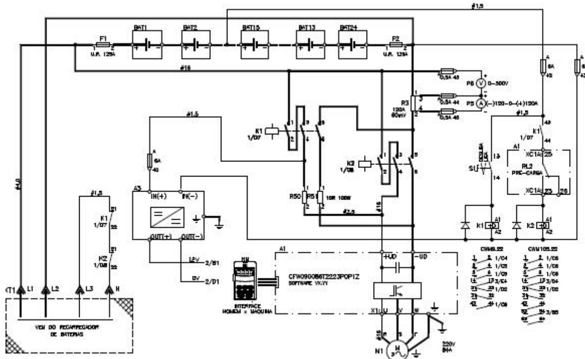
Figura 45 - Circuito elétrico do sistema de propulsão
