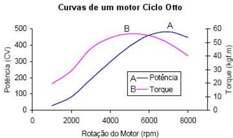
Figura 15 - Curvas de torque, potência de um motor ciclo Otto
