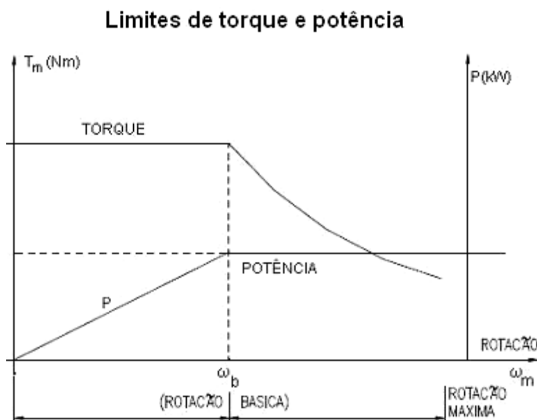
Figura 18 - Envoltória de desempenho do veículo (primeiro quadrante T_m > 0 e \omega_m > 0 )
