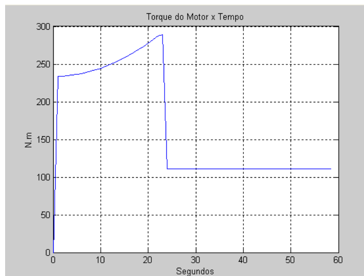
Figura 40 - Torque no motor, em N.m, versus tempo referente ao item 3.7.4
