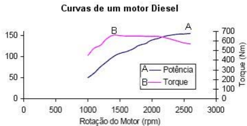
Figura 14 - Curvas de torque, potência de um motor Diesel
