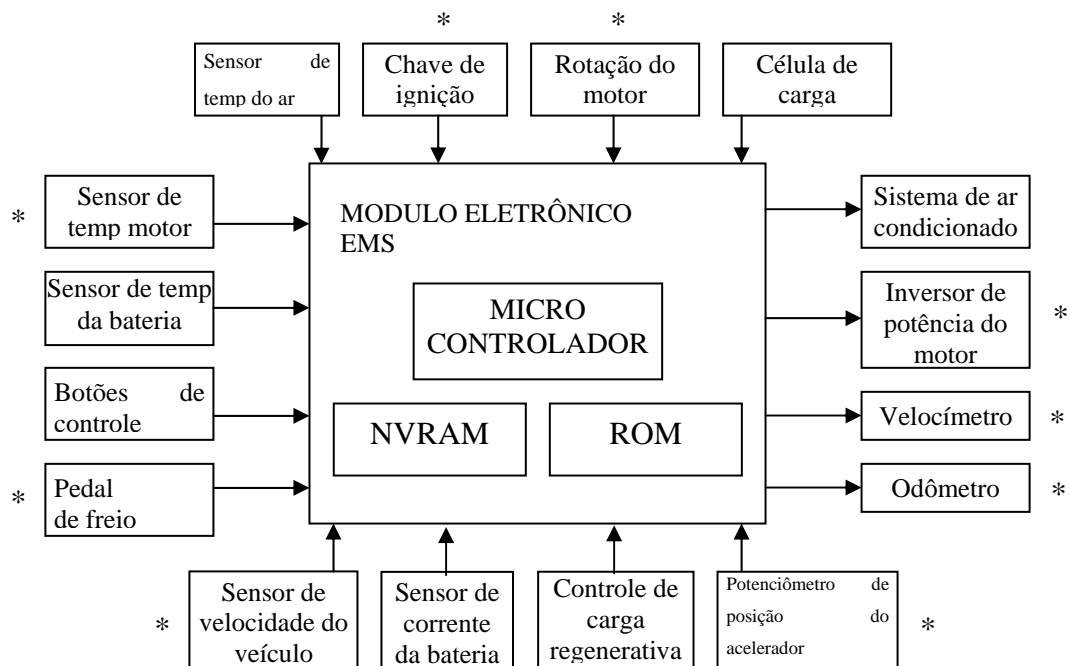
Figura 20 - EMS conjugado com um sistema de navegação elétrico
