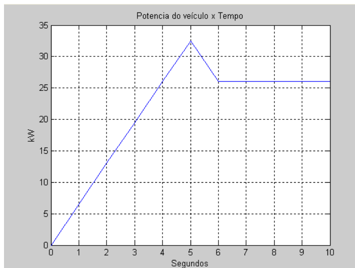
Figura 34 - Potência, em kw, desenvolvida pelo veículo versus tempo, referente ao item 3.7.3
