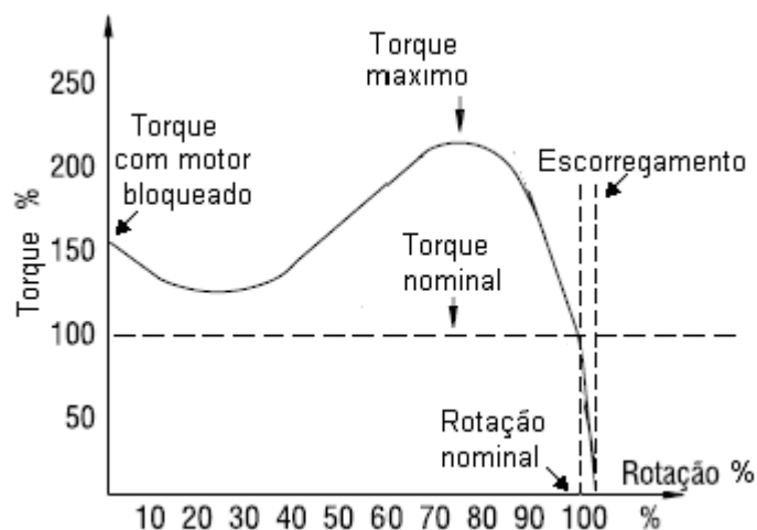
Figura 16 - Curva característica de torque de um motor de indução
