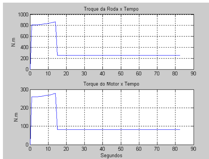
Figura 32 - Torque na roda e torque no motor em N.m, referente ao item 3.7.2
