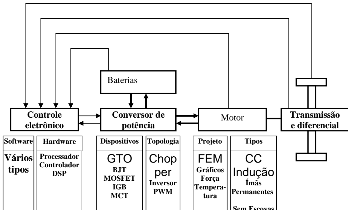
Figura 17 - Diagrama em bloco típico de um sistema de propulsão de veículo elétrico
