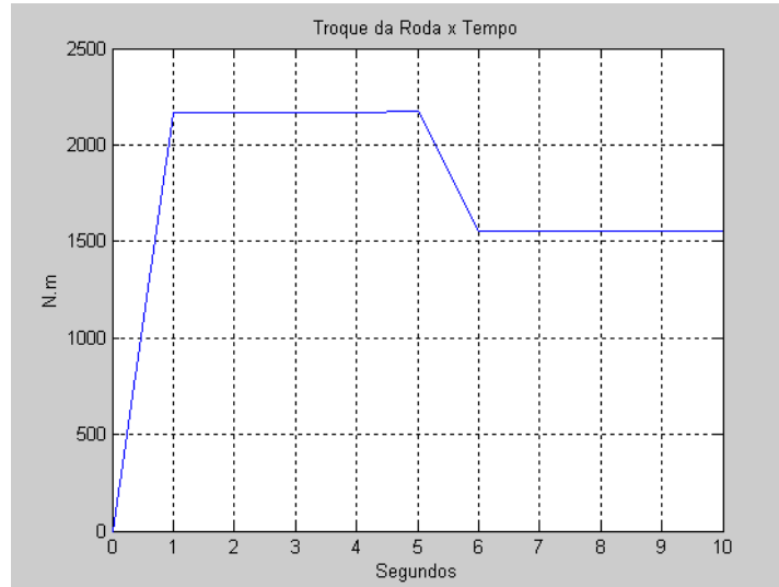
Figura 35 - Torque na roda, em N.m, versus tempo referente ao item 3.7.3
