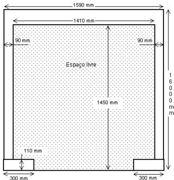
Figura 44 - Dimensões do compartimento interno da Kombi destinado ao banco de baterias e cargas a serem transportadas
