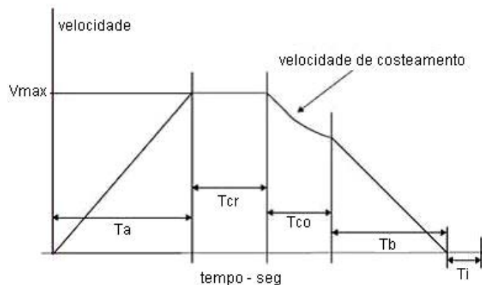
Figura 13 - Ciclo de testes SAE J227a
