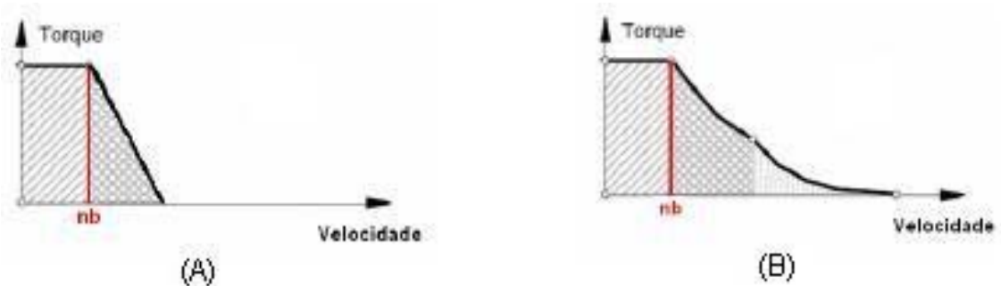
Figura 28 - (A) Curva de torque e velocidade dos motores com ímãs superficiais e (B) Curva de torque e velocidade dos motores com ímãs internos
