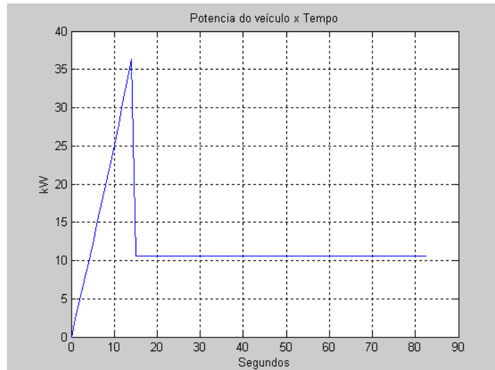
Figura 31 - Potência em kw desenvolvida pelo veículo, referente ao item 3.7.2
