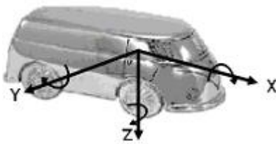
Figura 23 - Sistema de coordenadas SAE J 670, americano
