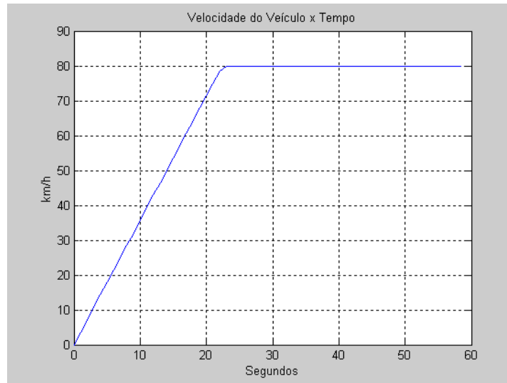
Figura 37 - Velocidade do veículo em km/h versus tempo referente ao item 3.7.4
