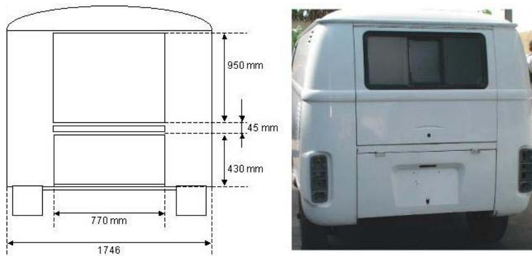
Figura 43 - Parte traseira da Kombi (altura total do solo até o teto – 1.912 mm)
