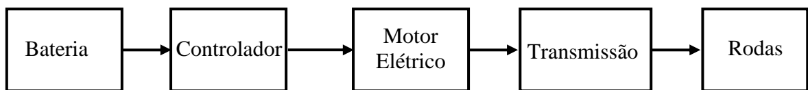
Figura 12 - Diagrama esquemático para determinação do motor de um veículo elétrico
