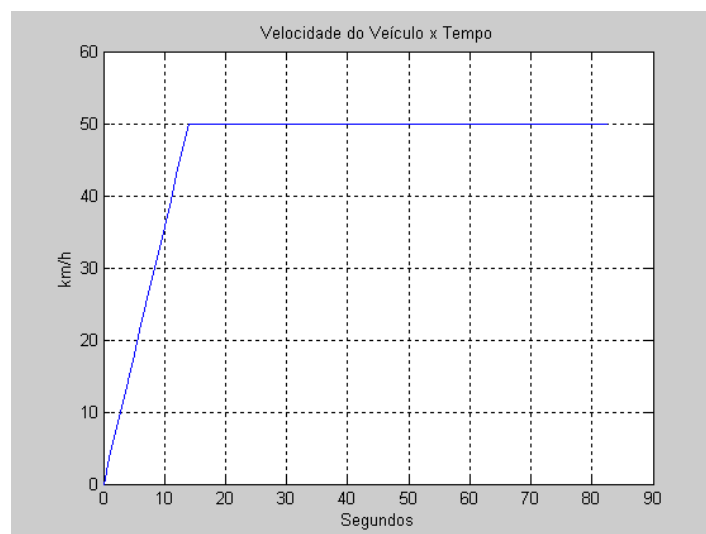
Figura 30 - Velocidade do veículo em km/h referente ao item 3.7.2
