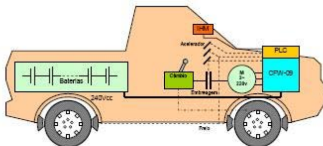
Figura 5 - Saveiro Elétrico WEG Fonte: WEG Indústrias S.A. – Automação
