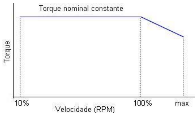
Figura 29 - Curva de torque e velocidade de um motor síncrono controlado por inversor
