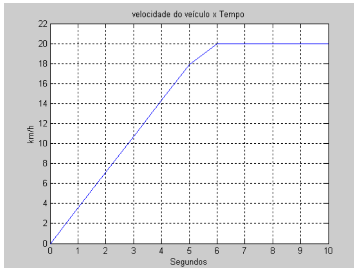
Figura 33 - Velocidade do veículo, em km/h, versus tempo, referente ao item 3.7.3
