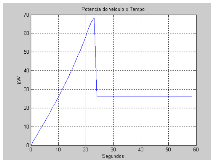
Figura 38 - Potência em kw desenvolvida pelo veículo versus tempo referente ao item 3.7.4
