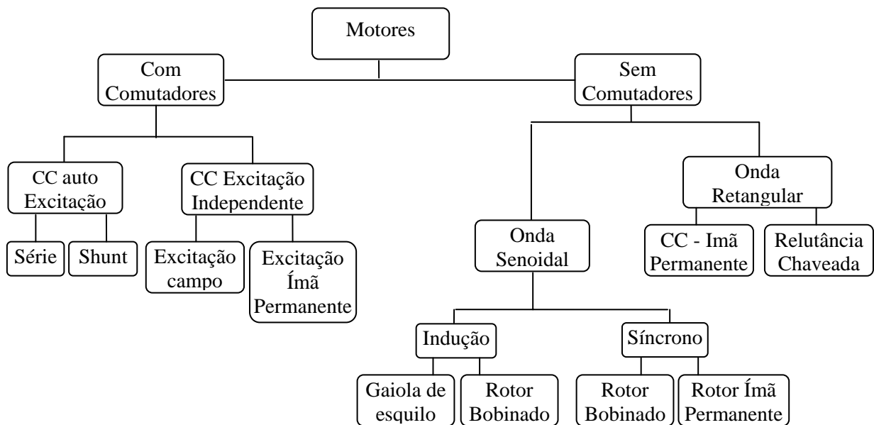
Figura 19 - Classificação típica dos motores elétricos para propulsão EV
