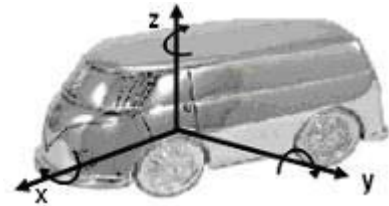
Figura 24 - Sistema de coordenadas ISO 4130 e DIN 70000, europeu.
