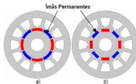
Figura 27 - Motor com ímãs superficiais (a) ou ímãs internos (b) no rotor.
