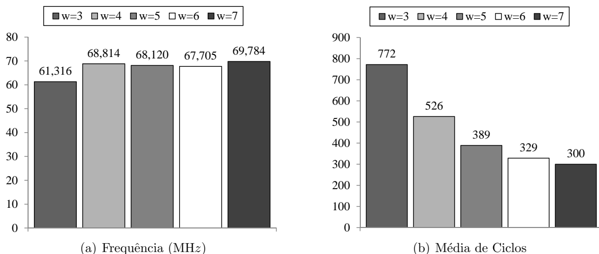
Figura 31: Resultados de tempo para variações em w .
