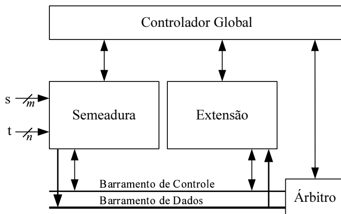
Figura 4: Macro-Arquitetura: Divisão pelas etapas do algoritmo
