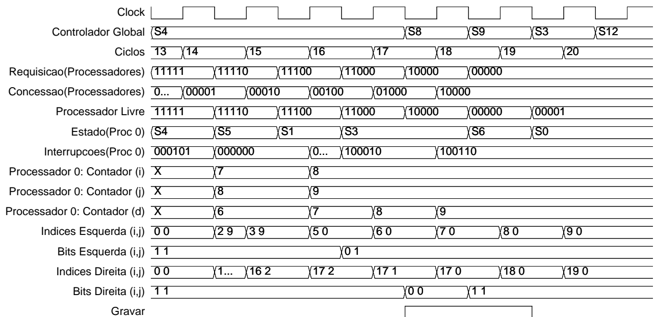
Figura 27: Índices atualizados e término da extensão
