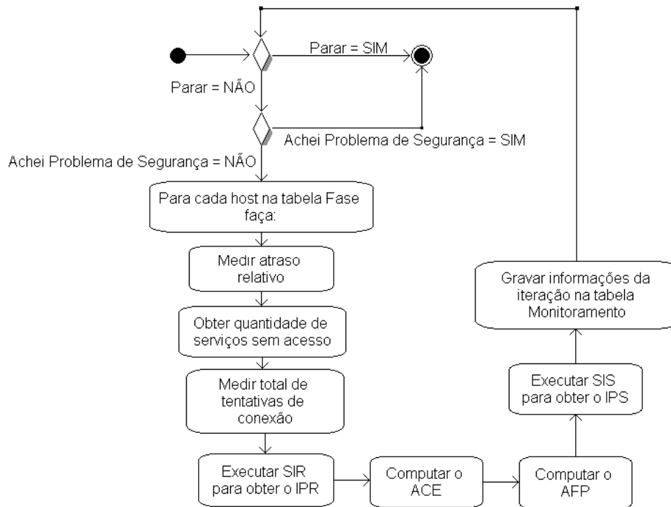
Figura 28 – Algoritmo de Monitoramento do Gestor de Software na Nuvem
