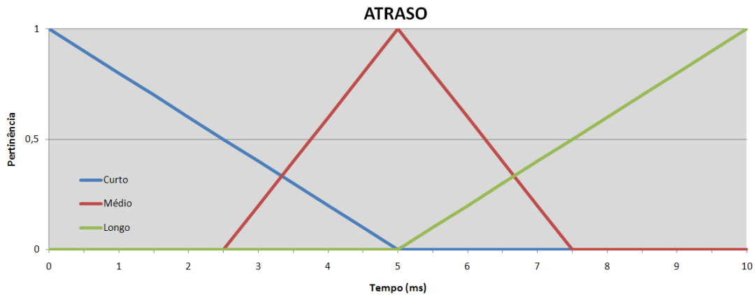
Figura 21 – Funções de Pertinência dos Termos da Variável Linguística ATRASSO.
