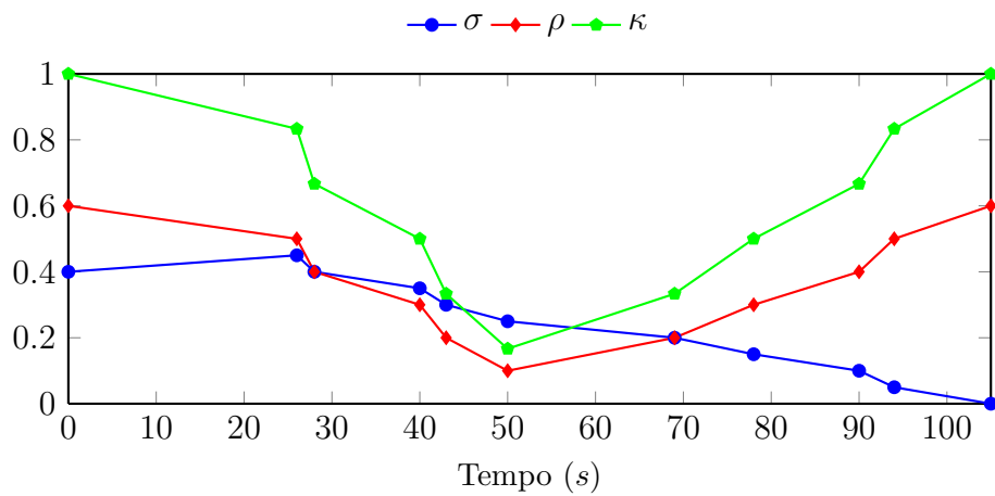
Figura 69: Evolução temporal da experiência 16: enxame de 20 Kilobots , 2 classes e 6 cargas estáticas iniciais
