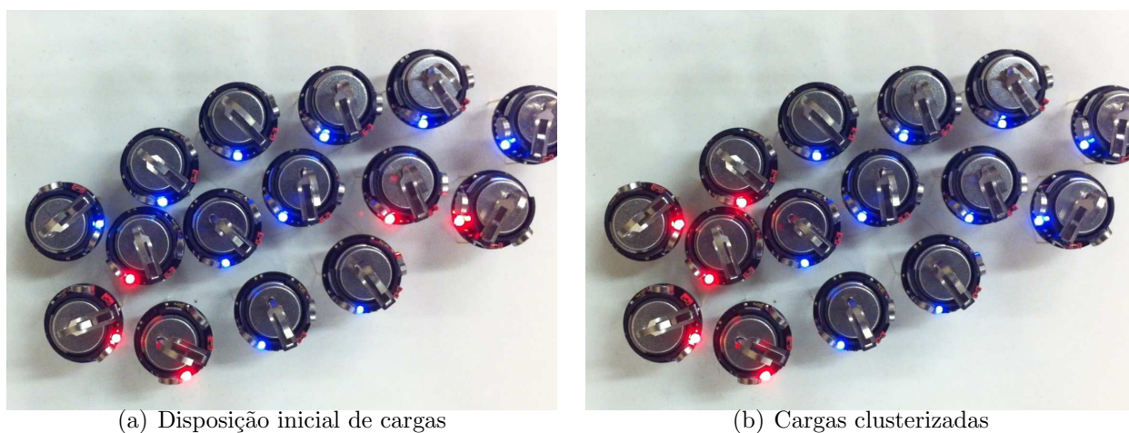
Figura 52: Experiência 8: enxame de 15 Kilobots , 2 classes e 5 cargas estáticas iniciais
