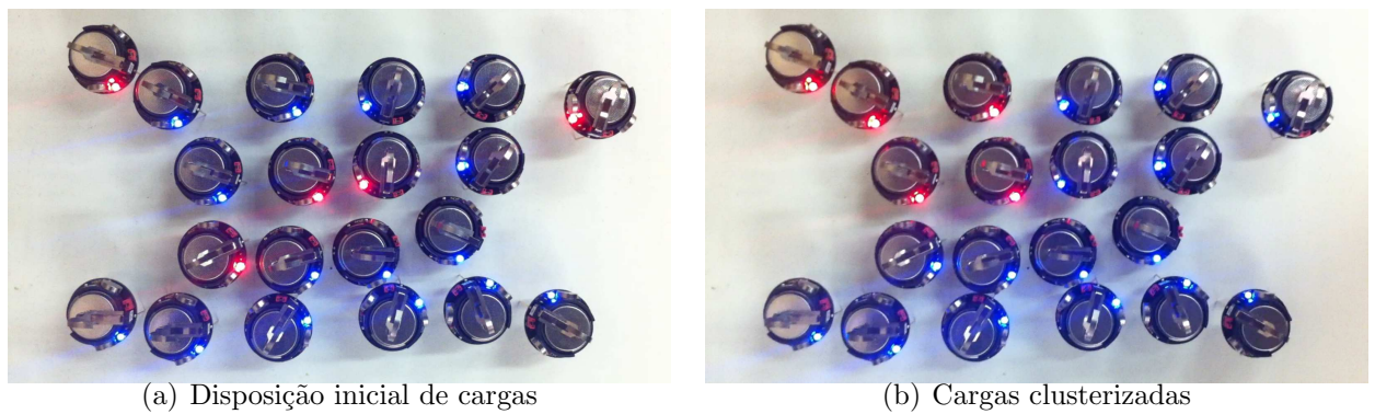
Figura 66: Experiência 15: enxame de 20 Kilobots , 2 classes e 5 cargas estáticas iniciais
