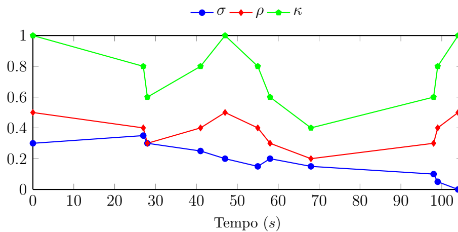
Figura 67: Evolução temporal da experiência 15: enxame de 20 Kilobots , 2 classes e 5 cargas estáticas iniciais
