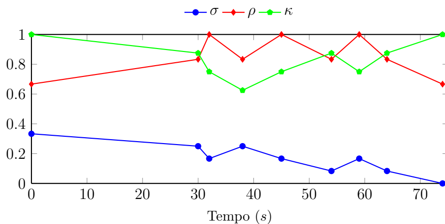
Figura 47: Evolução temporal da experiência 5: enxame de 12 Kilobots , 2 classes e 8 cargas estáticas iniciais
