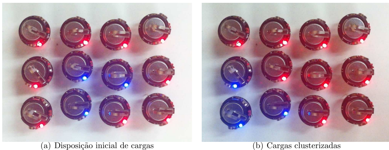
Figura 48: Experiência 6: enxame de 12 Kilobots , 2 classes e 9cargas estáticas iniciais
