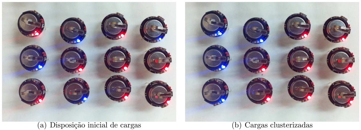
Figura 46: Experiência 5: enxame de 12 Kilobots , 2 classes e 8 cargas estáticas iniciais
