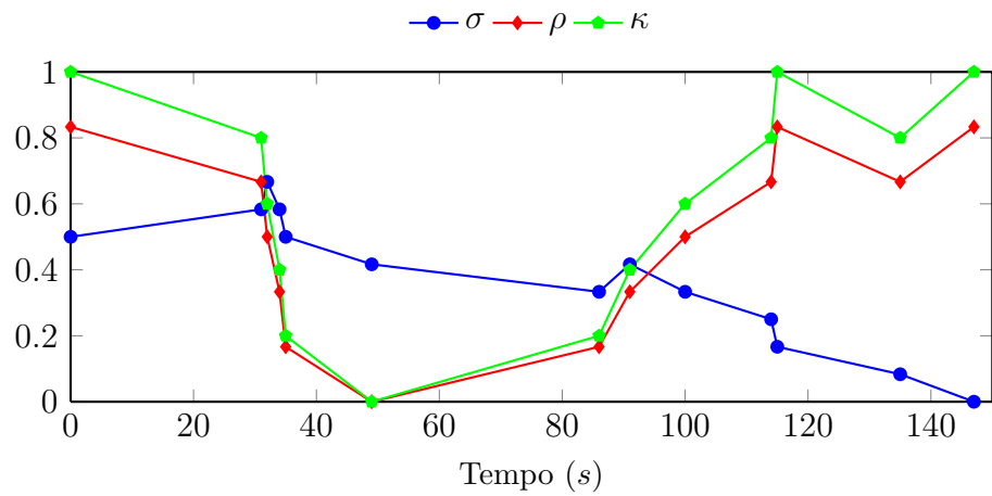
Figura 45: Evolução temporal da experiência 4: enxame de 12 Kilobots , 2 classes e 5 cargas estáticas iniciais
