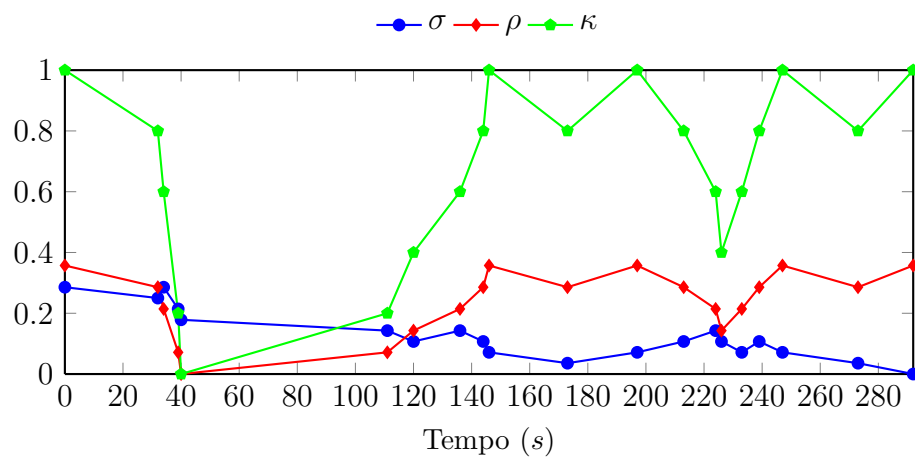
Figura 79: Evolução temporal da experiência 21: enxame de 28 Kilobots , 2 classes e 5 cargas estáticas iniciais
