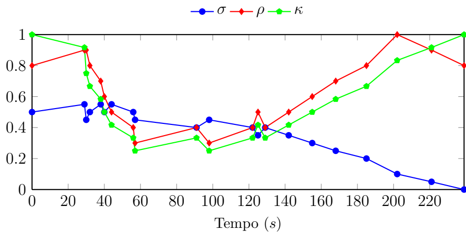
Figura 75: Evolução temporal da experiência 19: enxame de 20 Kilobots , 2 classes e 12 cargas estáticas iniciais
