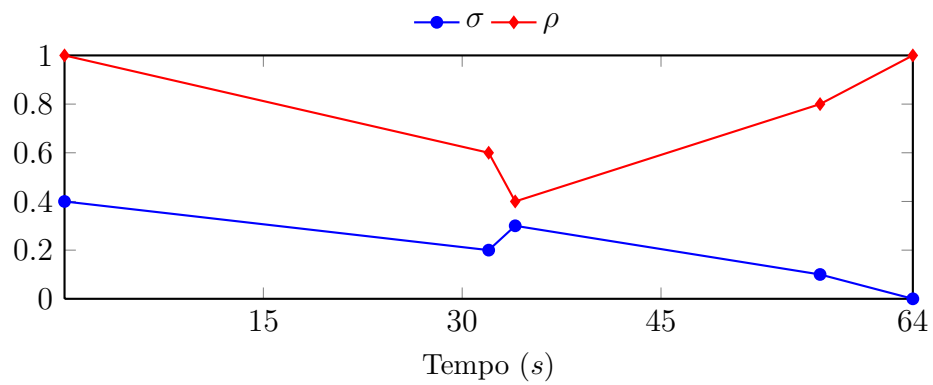
Figura 41: Evolução temporal da experiência 2: enxame de 10 Kilobots , 2 classes e 5 cargas estáticas iniciais
