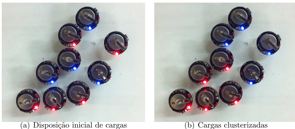
Figura 38: Experiência 1: enxame de 9 Kilobots , 2 classes e 5 cargas estáticas iniciais
