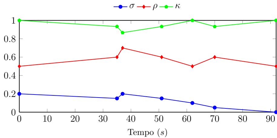
Figura 77: Evolução temporal da experiência 20: enxame de 20 Kilobots , 2 classes e 15 cargas estáticas iniciais
