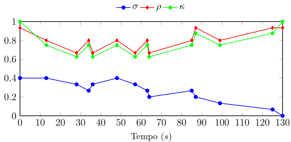
Figura 55: Evolução temporal da experiência 9: enxame de 15 Kilobots , 2 classes e 8 cargas estáticas iniciais
