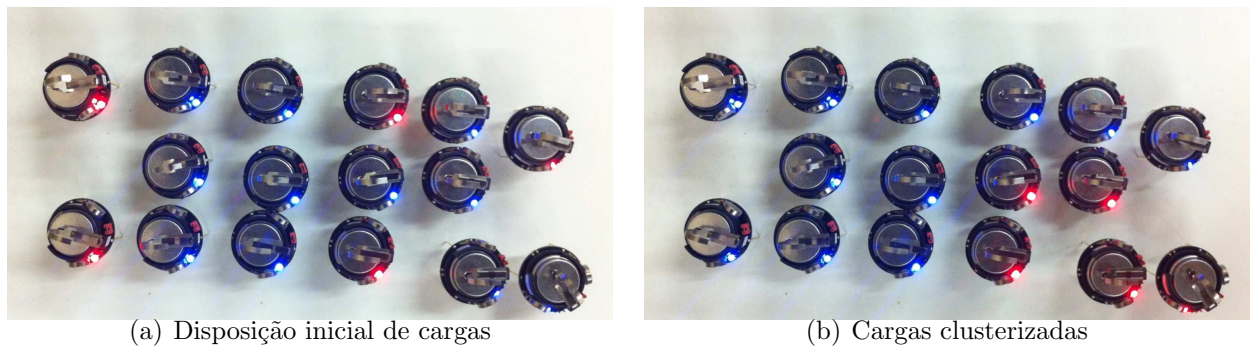
Figura 56: Experiência 10: enxame de 16 Kilobots , 2 classes e 5 cargas estáticas iniciais
