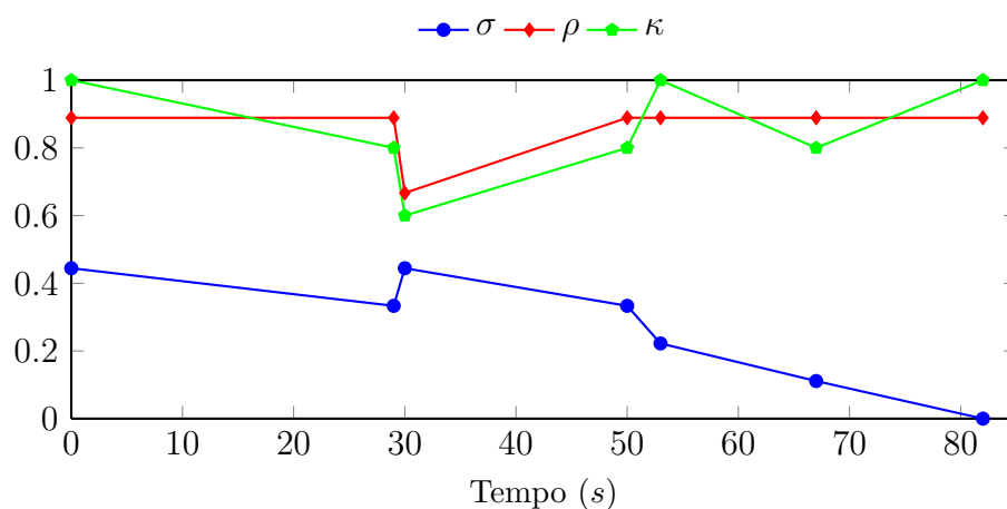
Figura 39: Evolução temporal da experiência 1: enxame de 9 Kilobots , 2 classes e 5 cargas estáticas iniciais
