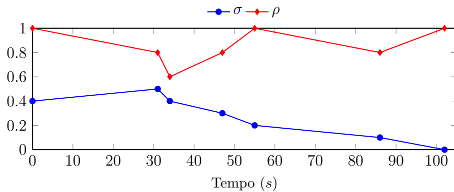
Figura 43: Evolução temporal da experiência 3: enxame de 10 Kilobots , 2 classes e 5 cargas estáticas iniciais
