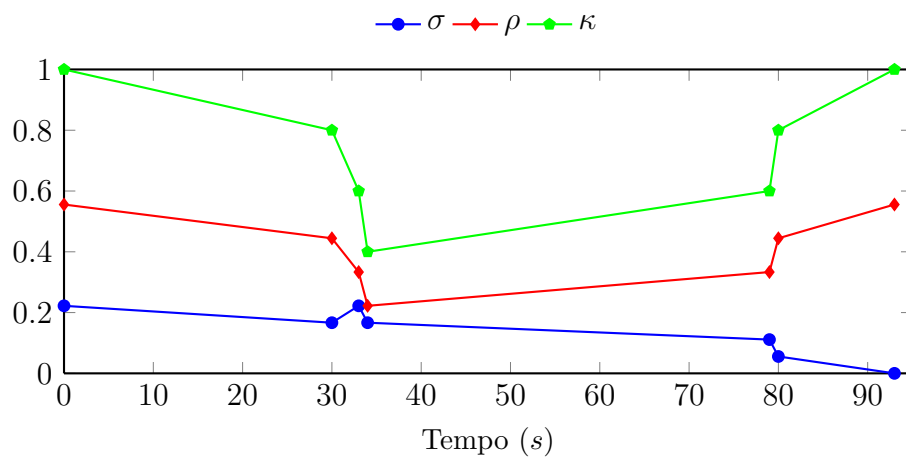
Figura 63: Evolução temporal da experiência 13: enxame de 18 Kilobots , 2 classes e 5 cargas estáticas iniciais
