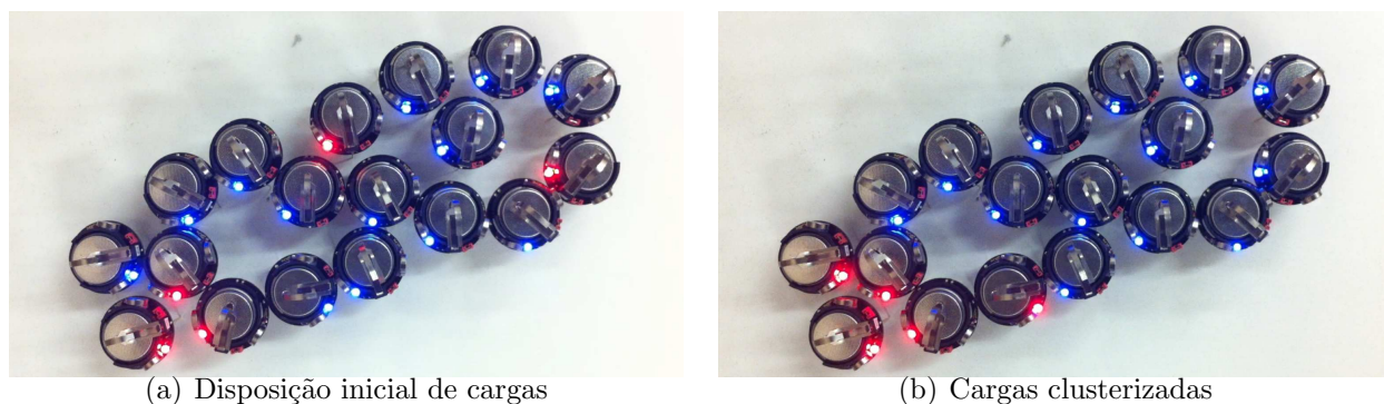
Figura 62: Experiência 13: enxame de 18 Kilobots , 2 classes e 5 cargas estáticas iniciais
