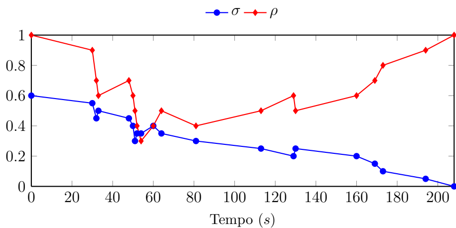
Figura 73: Evolução temporal da experiência 18: enxame de 20 Kilobots , 2 classes e 10 cargas estáticas iniciais
