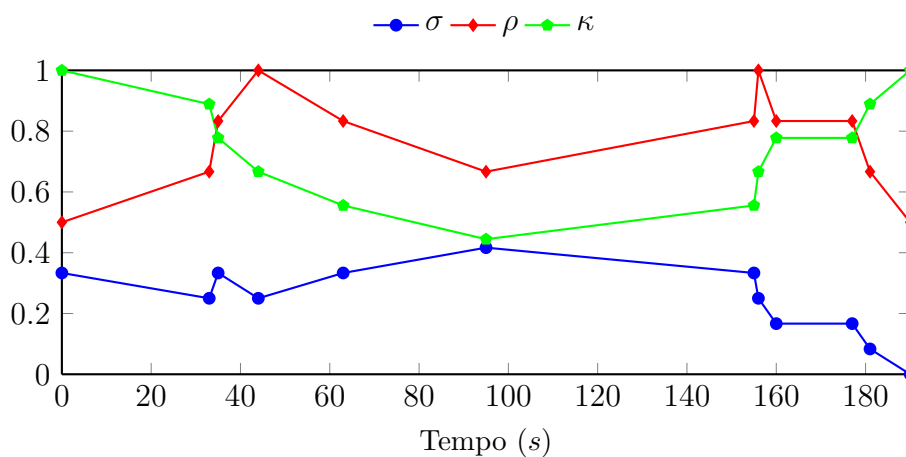
Figura 49: Evolução temporal da experiência 6: enxame de 12 Kilobots , 2 classes e 9 cargas estáticas iniciais
