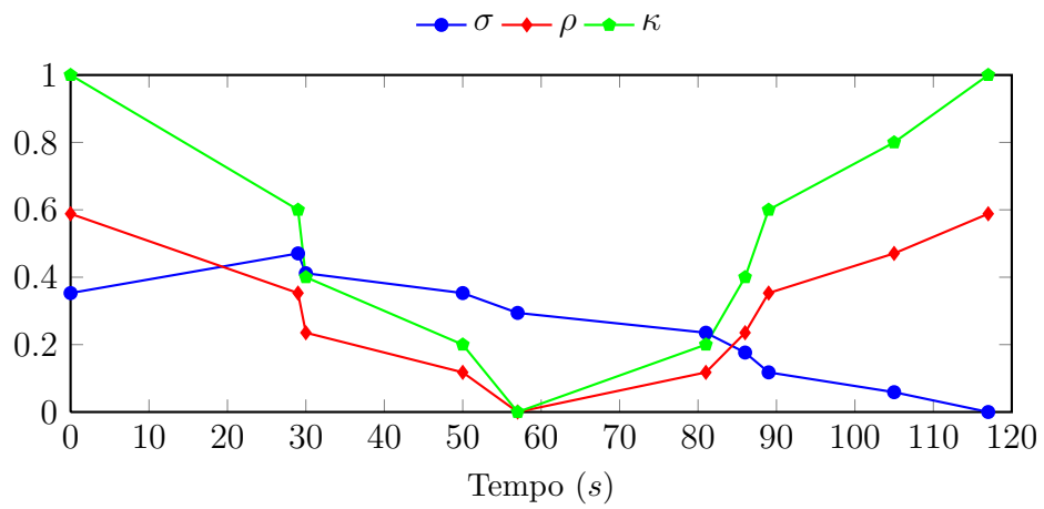
Figura 59: Evolução temporal da experiência 11: enxame de 17 Kilobots , 2 classes e 5 cargas estáticas iniciais
