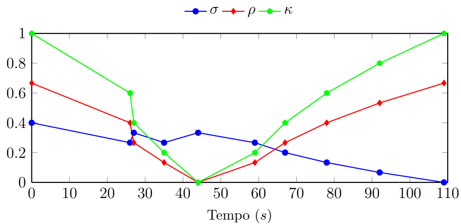
Figura 53: Evolução temporal da experiência 8: enxame de 15 Kilobots , 2 classes e 5 cargas estáticas iniciais
