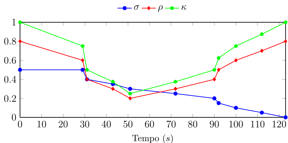
Figura 71: Evolução temporal da experiência 17: enxame de 20 Kilobots , 2 classes e 8 cargas estáticas iniciais
