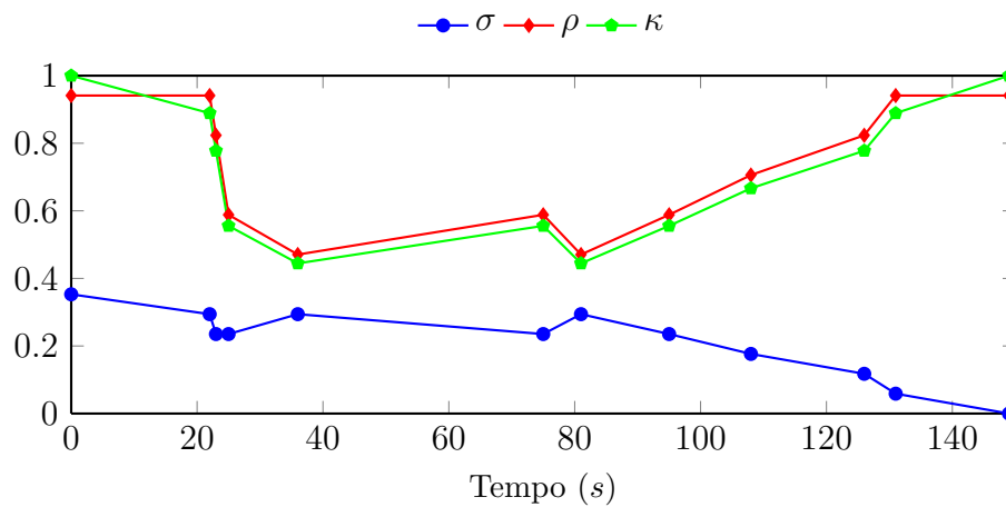
Figura 61: Evolução temporal da experiência 12: enxame de 17 Kilobots , 2 classes e 9 cargas estáticas iniciais
