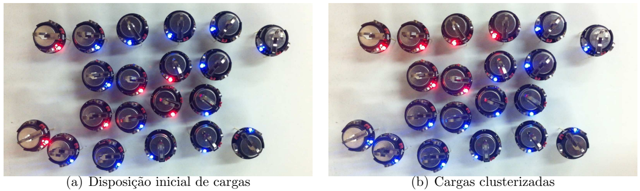
Figura 68: Experiência 16: enxame de 20 Kilobots , 2 classes e 6 cargas estáticas iniciais
