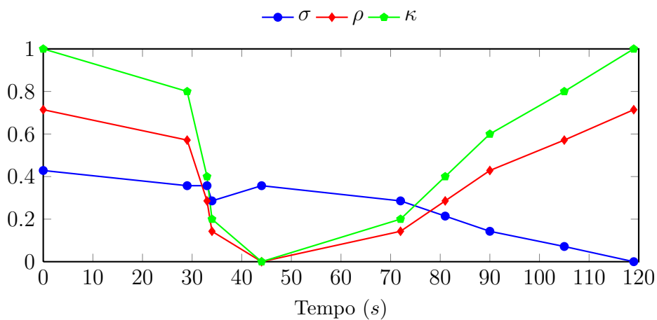
Figura 51: Evolução temporal da experiência 7: enxame de 14 Kilobots , 2 classes e 5 cargas estáticas iniciais
