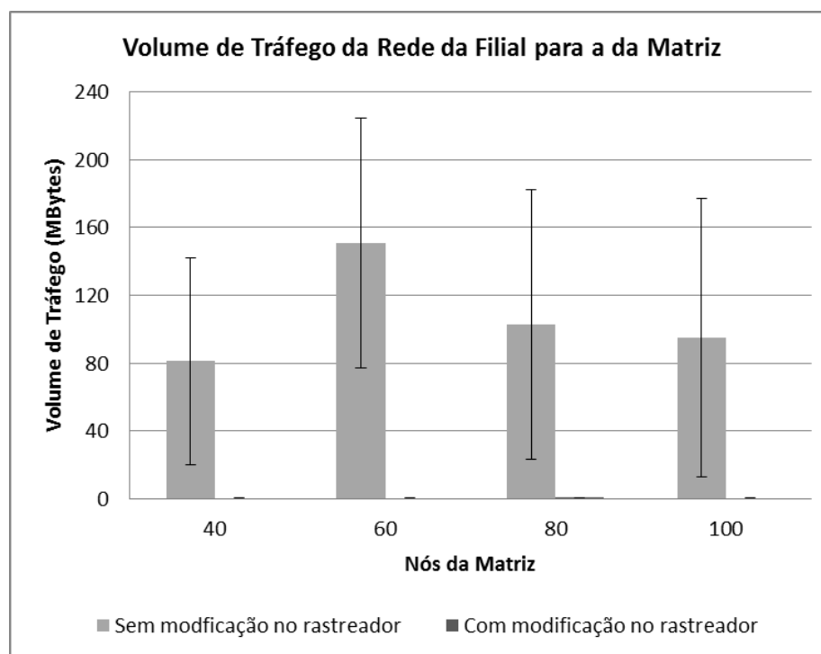
Figura 10 - Volume de tráfego da rede da Filial para a da Matriz – 155 Mbps.
