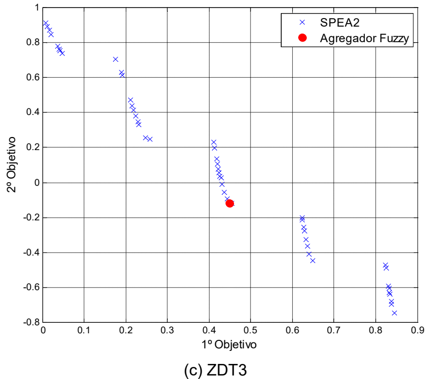
Figura 40 - Resultados obtidos para três problemas ZDT com 5 variáveis.
