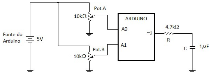
Figura 64 – Circuito implementado.
