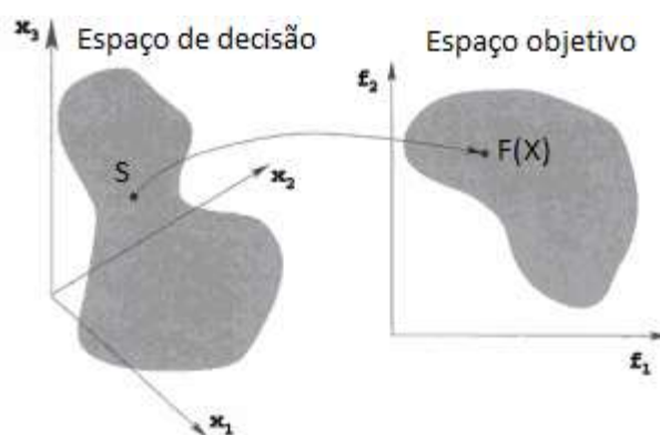
Figura 12 - Representação do espaço de decisão e espaço objetivo.
