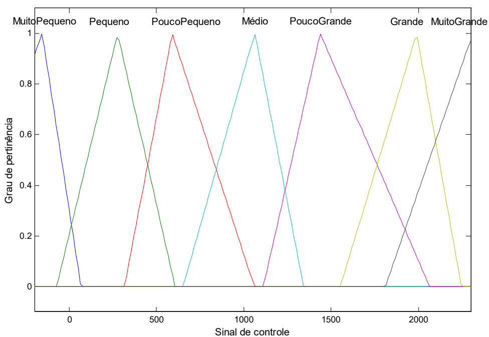
Figura 63 - Funções de pertinência para a saída 'Sinal de Controle'.
