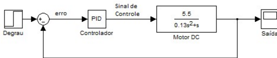
Figura 56 – Diagrama do sistema de controle para servossistema do motor CC.
