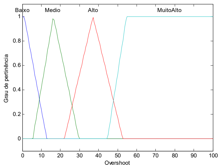
Figura 48 – Função de pertinência da variável de entrada Overshoot.
