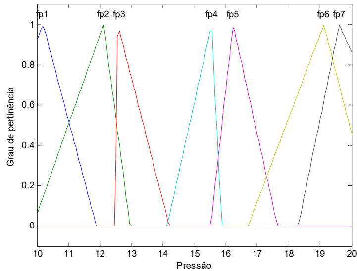
Figura 44 – Funções de pertinência do melhor resultado para o problema Plastic .
