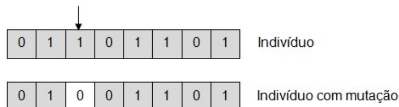
Figura 9 – Operador de mutação simples.
