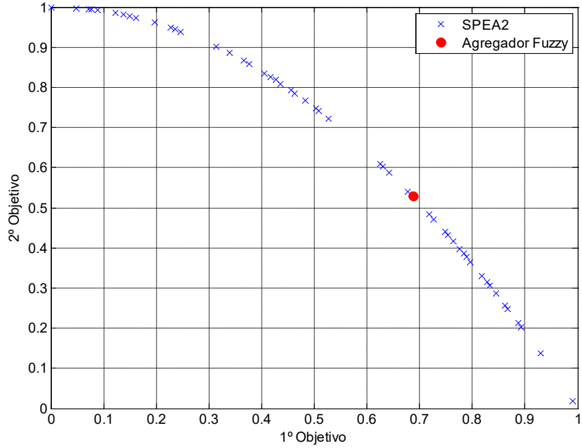
(b) ZDT2
