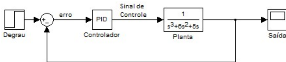
Figura 53 – Diagrama do sistema de controle de 3ª ordem.
