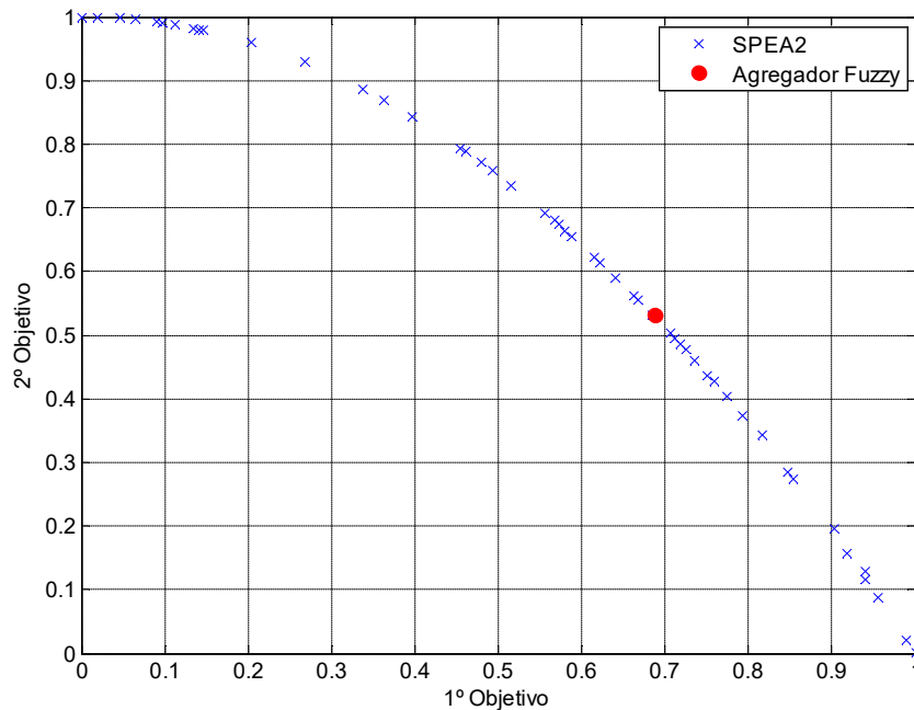
(b) ZDT2
