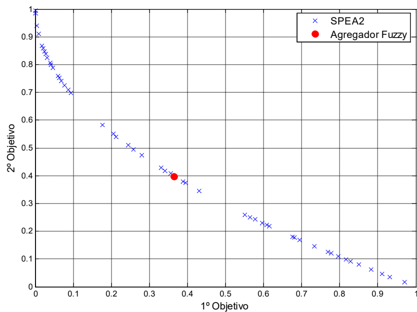
(a) ZDT1
