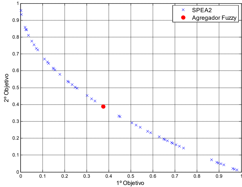
(a) ZDT1
