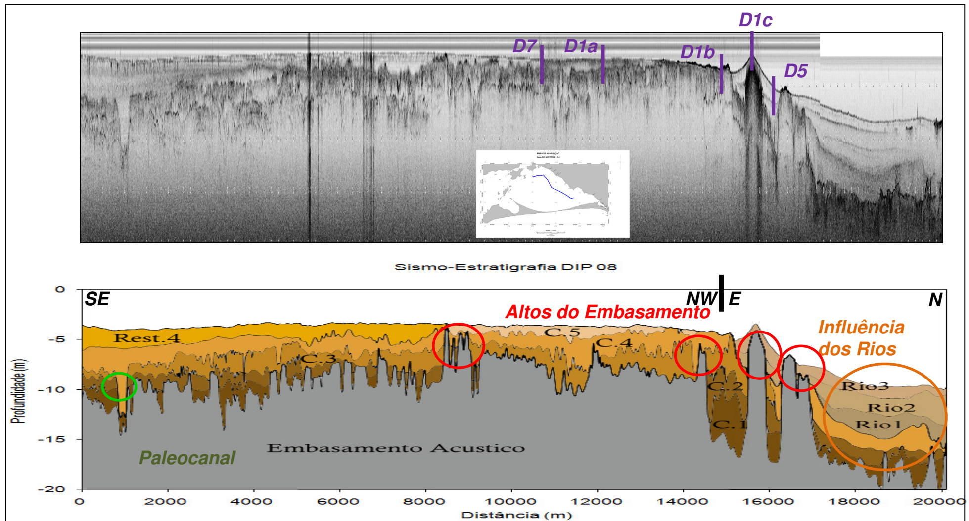
Figura 39 - Dado bruto e interpretação dos horizontes sísmicos do perfil D8. O círculo em verde mostra o padrão de paleocanal. Os círculos em vermelho mostram os altos do embasamento acústico, e o laranja, a influência dos Rios Guandu e Itaguaí. O traçado em preto indica a mudança de direção do perfil. Já o traçado roxo mostra o cruzamento com os perfis D1 (D1a, D1b e D1c), D5 e D7.
