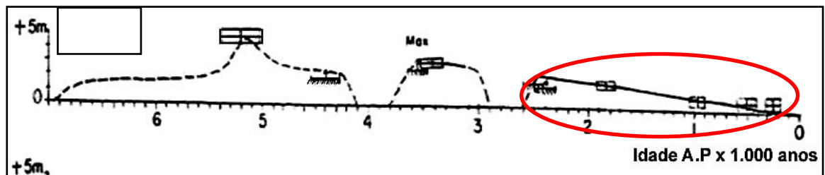
Figura 50 - Curva de variação do nível relativo do mar nos últimos 7.000 anos, destacando o período de deposição da Camada 5.
