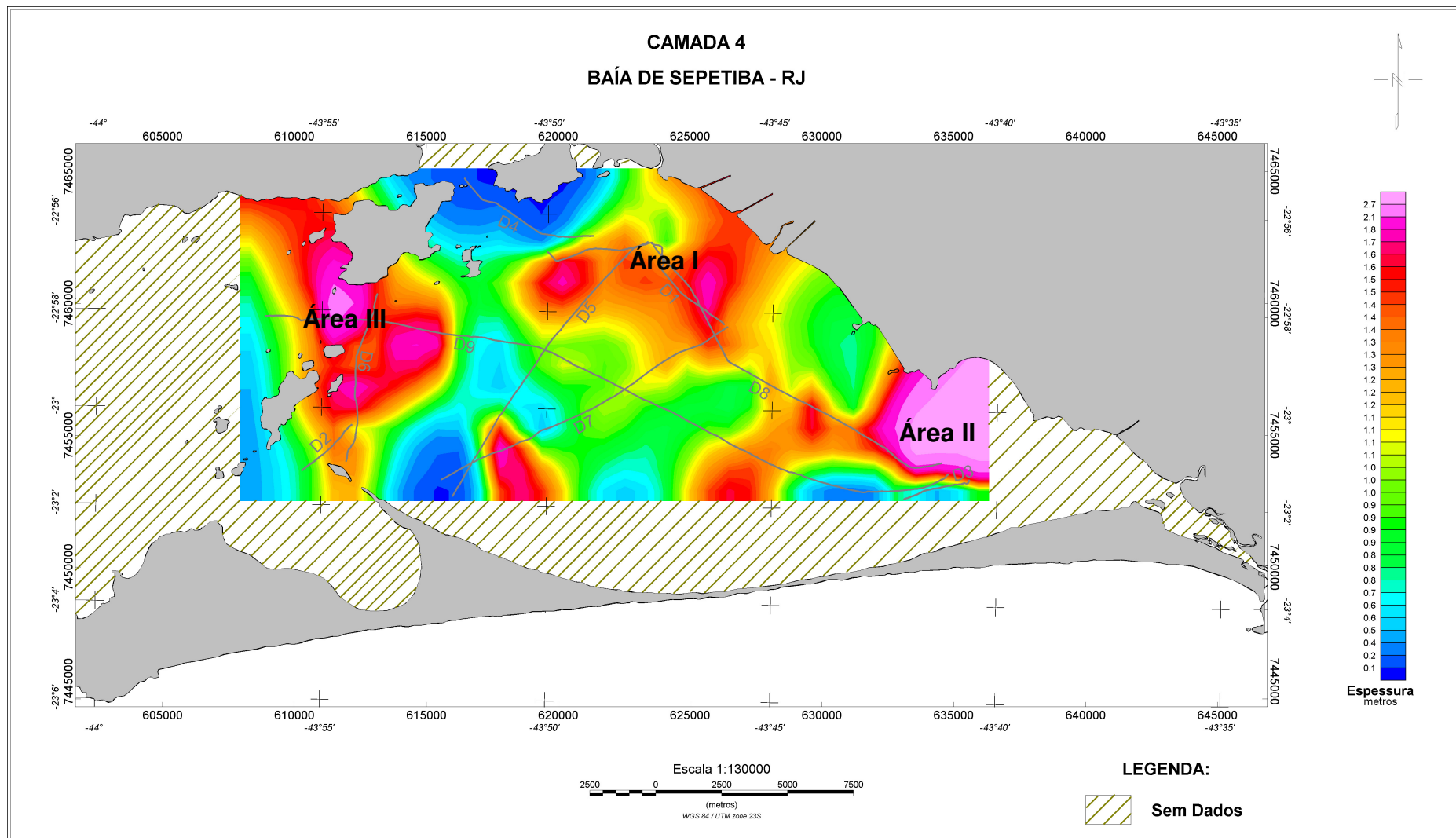
Figura 49 - Mapa de Isópacas da Camada 4. Em tons de azul, as menores espessuras e em tons de rosa, as maiores. Posicionamento das linhas sísmicas em cinza.
