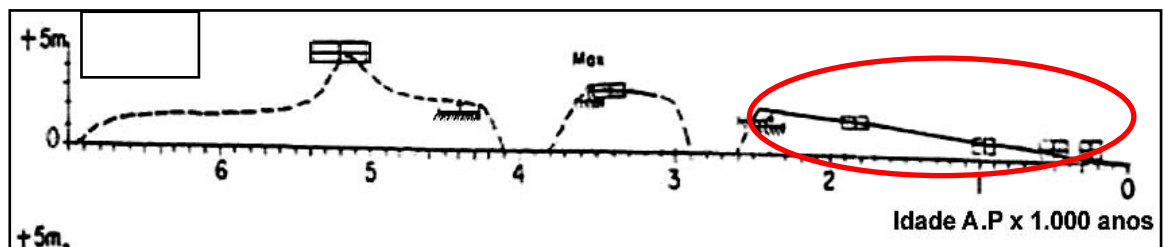
Figura 54 - Curva de variação do nível relativo do mar nos últimos 7.000 anos, destacando o período de deposição das Camadas Rio 1, Rio 2 e Rio 3.
