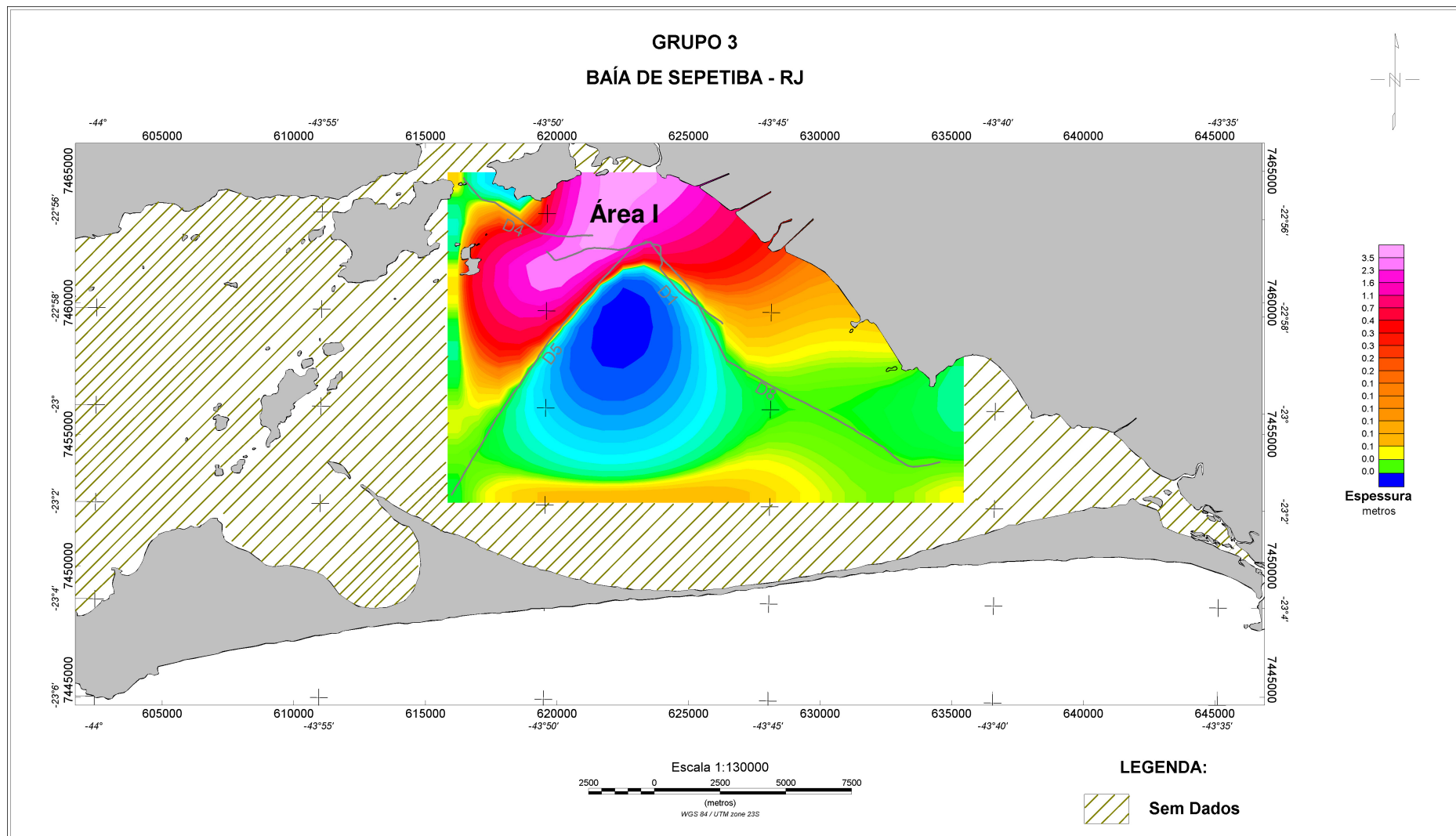
Figura 55 - Mapa de Isópacas do Grupo 3. Em tons de azul, as menores espessuras e em tons de rosa, as maiores. Posicionamento das linhas sísmicas em cinza.
