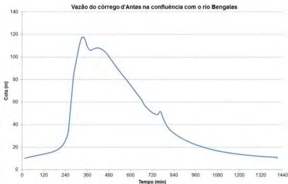
Figura 69 – Hidrograma de cheia do córrego d'Antas para a chuva com 25 anos de tempo de recorrência, na confluência com o rio Bengalas.
