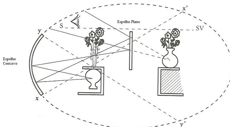
Figura 2 - Esquema simplificado de dois espelhos
