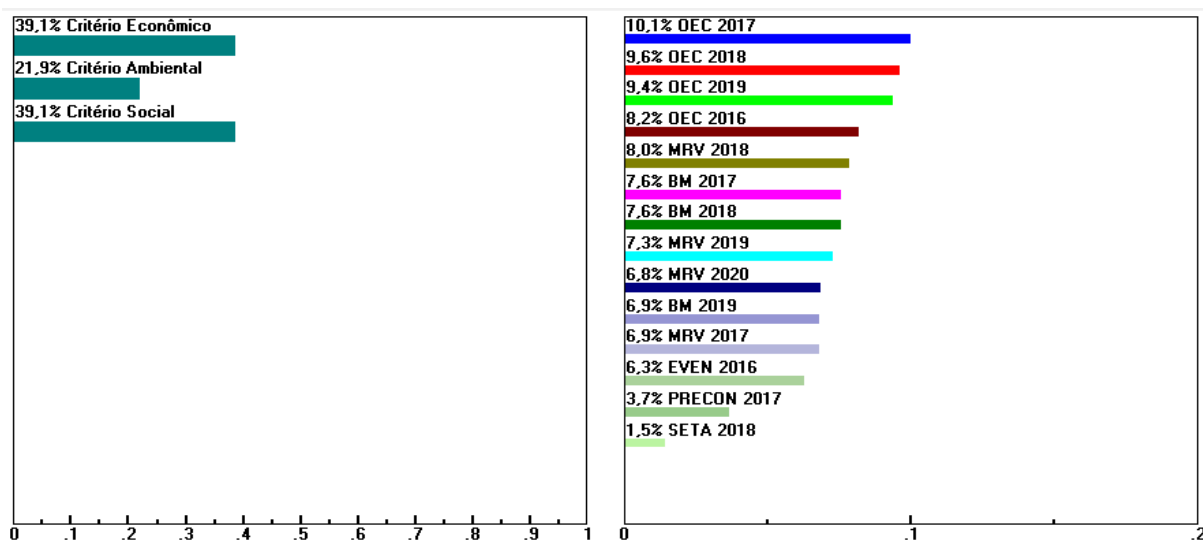
Figura 7 - Análise de sensibilidade (critério ambiental)
