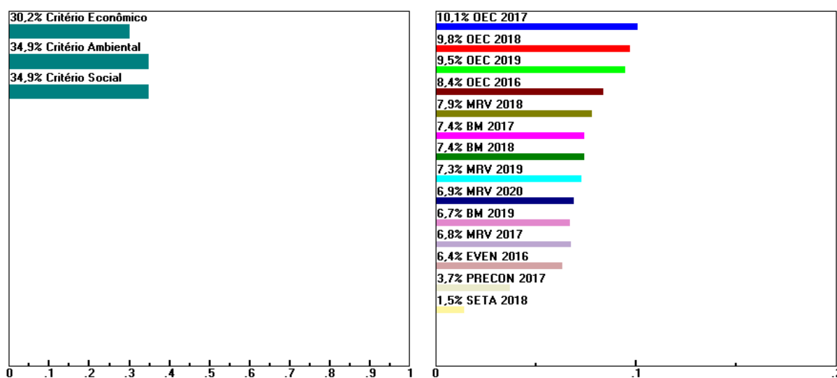
Figura 6 - Análise de sensibilidade (critério econômico)
