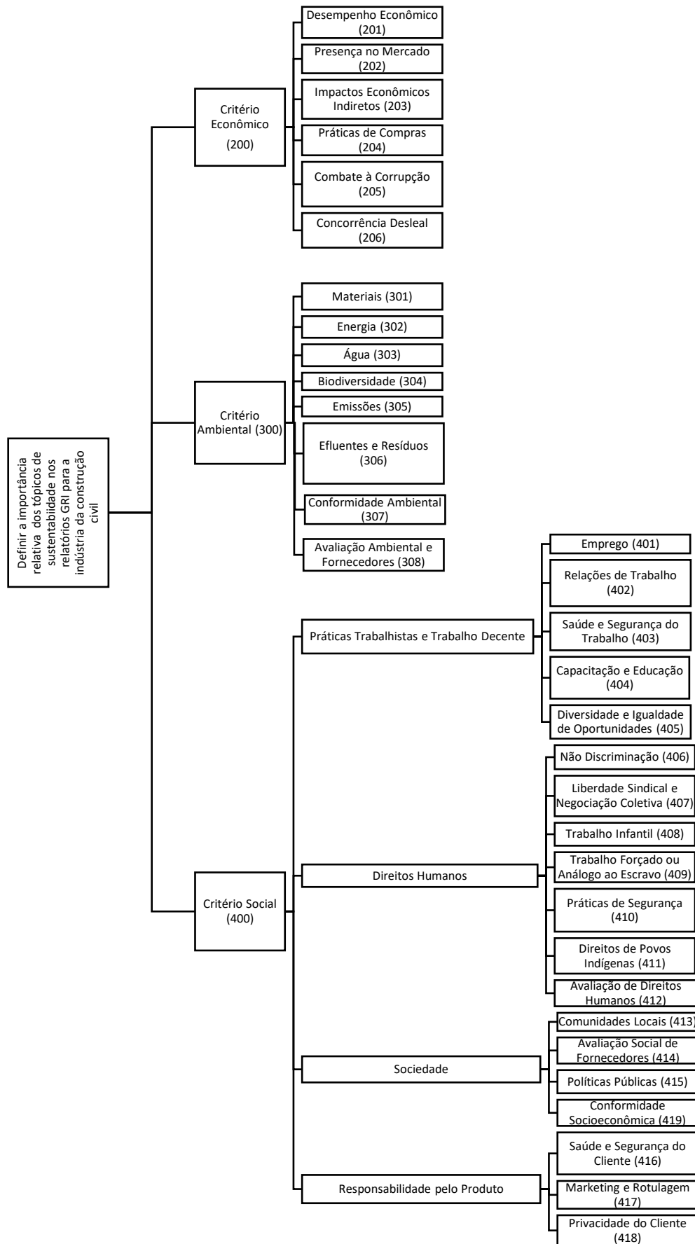
Figura 4 - Estrutura hierárquica do problema
