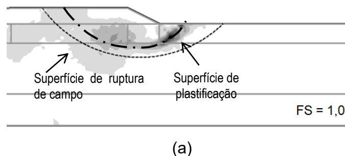
Figura 37 – Análises da ruptura do aterro com St^*=2,0 e malha de 5000 elementos (continua)
