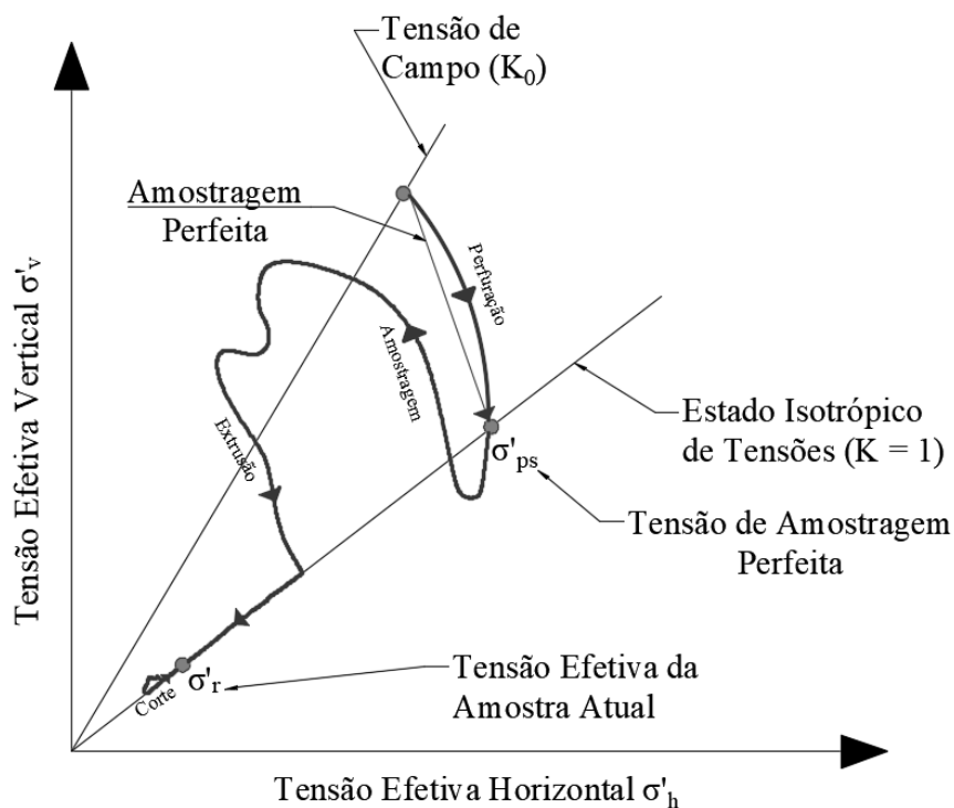
Figura 5 – Trajetória de tensões durante amostragem.
