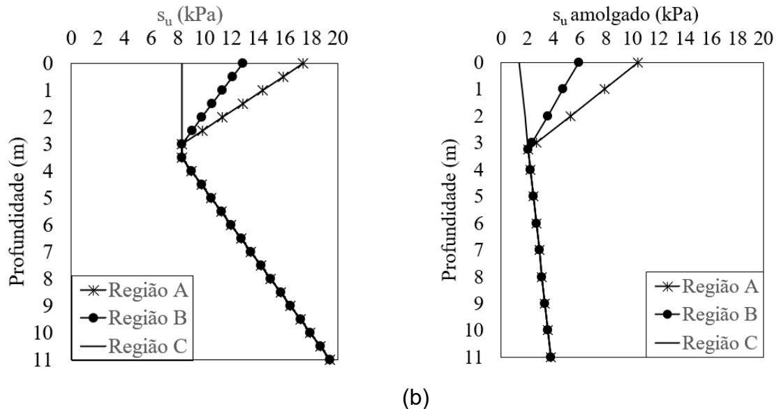
Figura 31 - Perfil de s_u representativo de Sarapu /RJ considerando-se ganho de resist ncia devido a dissip  o de poropress o na crosta superficial.
