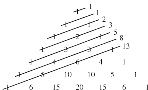
Figura 14 - Teorema das diagonais invertidas do Triângulo de pascal.
