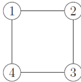
Figura 48 - Grafo C_4
