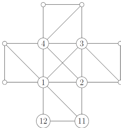
Figura 46 - Revertendo diagonais
