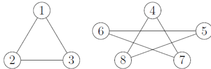
Figura 36 - Grafo das Bailarinas
