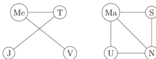
Figura 5 - Representação do problema 1.1.2
