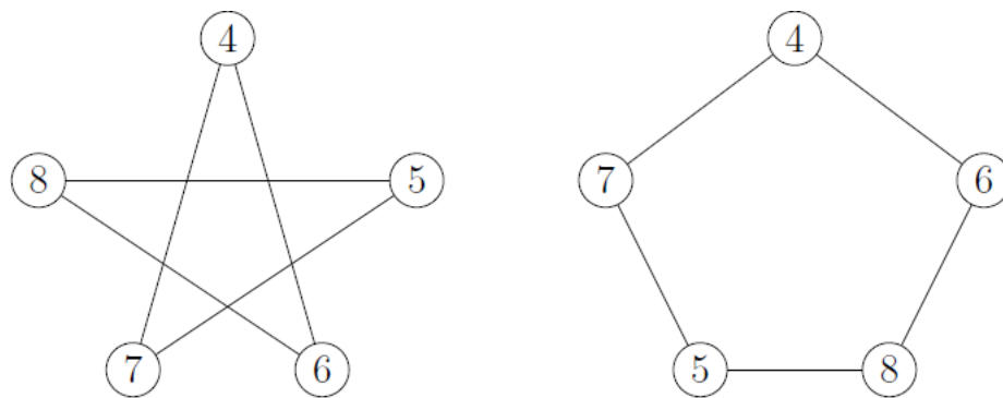
Figura 57 - Duas representações de C_5
