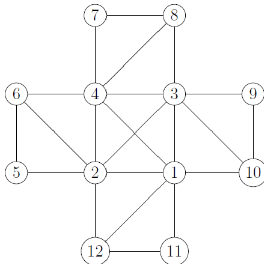
Figura 43 - Permutação Completa
