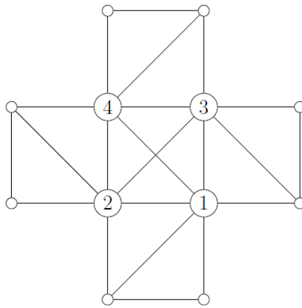
Figura 40 - Vértices \{1, 2, 3, 4\}
