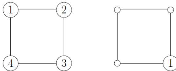
Figura 49 - Construindo um automorfismo de C_4
