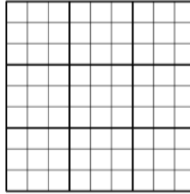
Figura 17 - Sudoku
