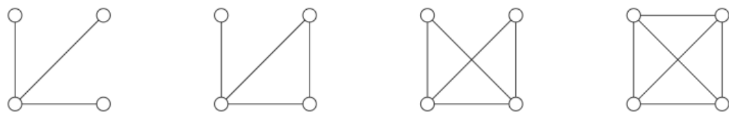
Figura 15 - Grafos para o caso n=4 e \Delta(G) = 3
