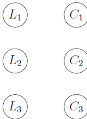
Figura 22 - Vértices
