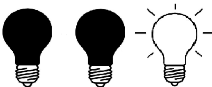
Figura 29 - Configuração impossível para as lâmpadas
