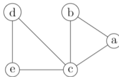
Figura 9 - Grafo de 5 vértices
