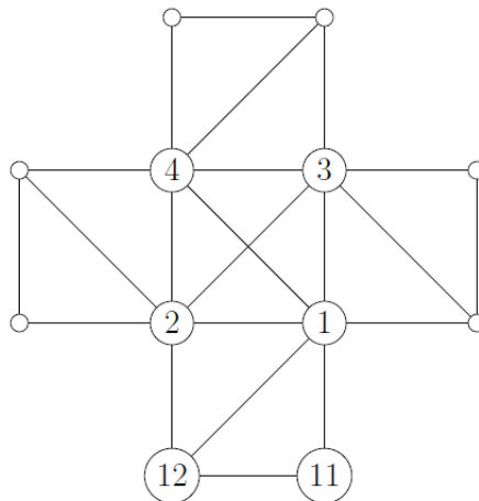
Figura 41 - Introdução dos vértices 11 e 12
