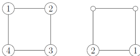
Figura 50 - Construindo um automorfismo de C_4
