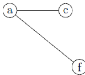
Figura 1 - Conexões de Alan
