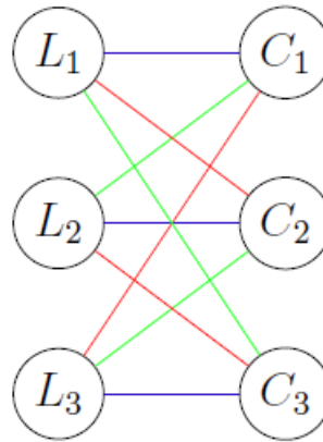
Figura 25 - Grafo
