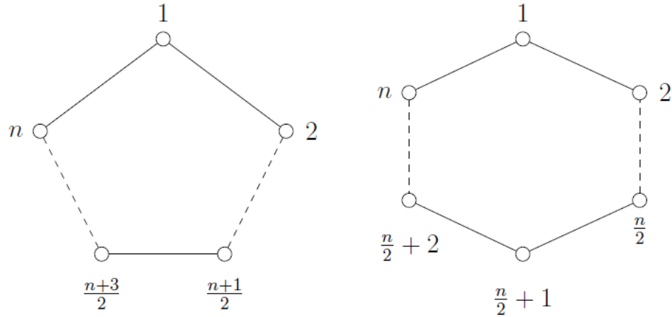
Figura 56 - C_n para os casos em que n é ímpar e par, respectivamente
