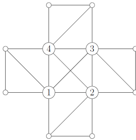
Figura 44 - Permutação (1423)
