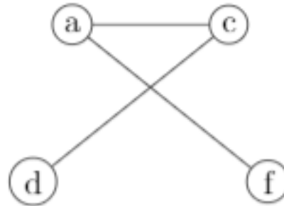
Figura 2 - Conexões de Alan, Carlos, Diego e Fuyuki
