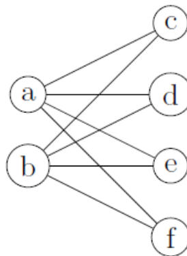
Figura 26 - Grafo K_{2,4}
