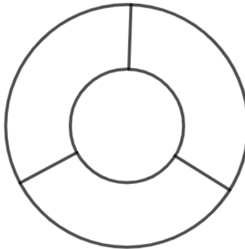
Figura 8 - Desenho
