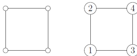
Figura 47 - Quadrado e seu grafo
