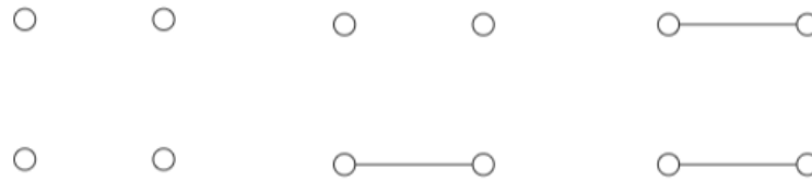
Figura 13 - Grafos para caso n = 4 , \Delta(G) = 0 e \Delta(G) = 1
