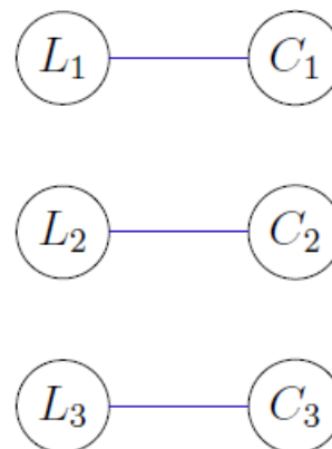
Figura 24 - Vértices e aresta
