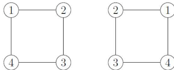
Figura 54 - Representação da transformação p_3
