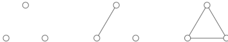
Figura 12 - Grafos para o caso n = 3
