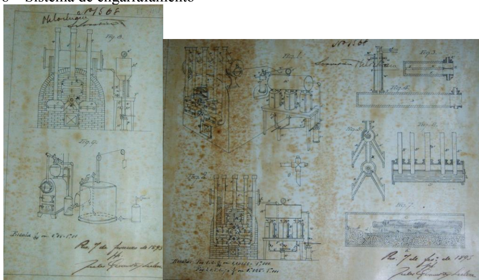
Figura 8 – Sistema de engarrafamento
