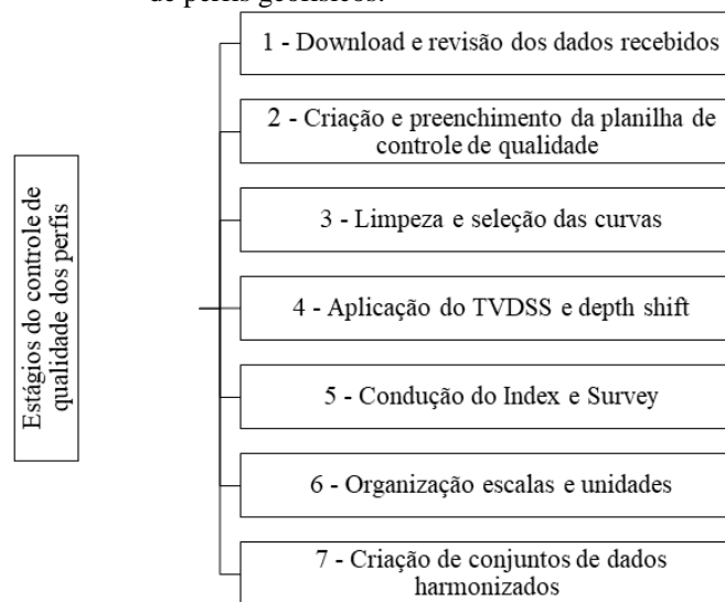
Figura 6 - Fluxograma do controle de qualidade dos dados de perfis geofísicos.
