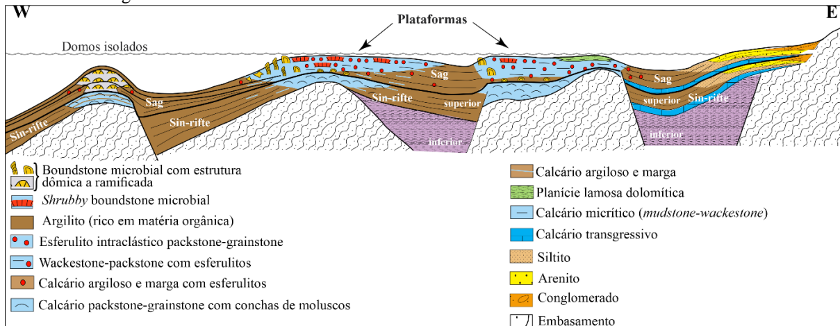
Figura 4 - Modelo estratigráfico esquemático do Pré-sal na Bacia de Kwanza, Angola: seção análoga à estratigrafia da Bacia de Santos.
