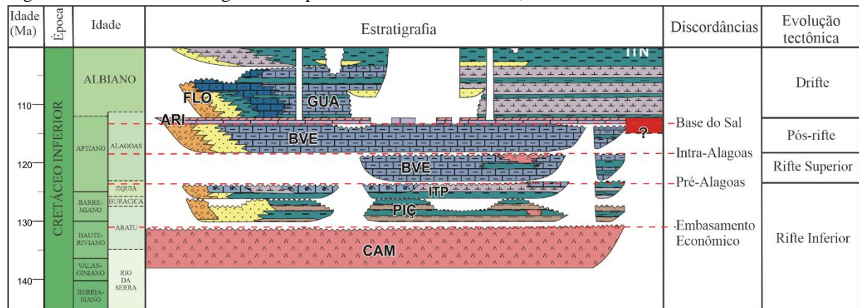
Figura 5 - Carta cronoestratigráfica simplificada da Bacia de Santos, detalhando o intervalo de interesse.
