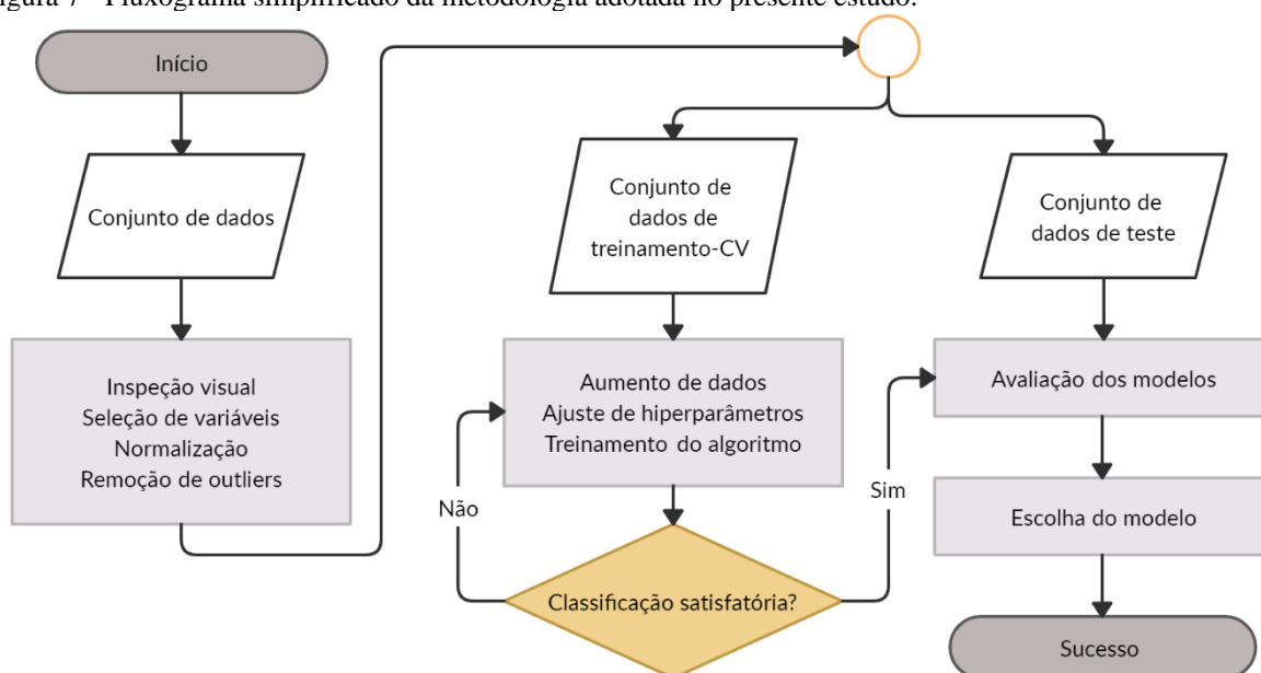
Figura 7 - Fluxograma simplificado da metodologia adotada no presente estudo.
