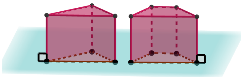
Figura 42 - Prisma Reto
