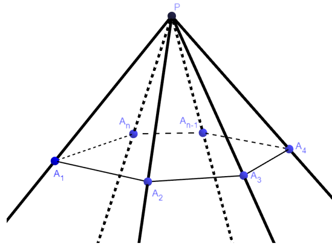
Figura 33 - Ângulo Poliédrico
