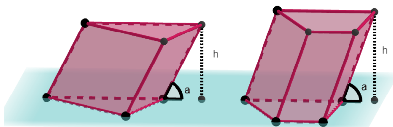
Figura 43 - Prisma Oblíquo
