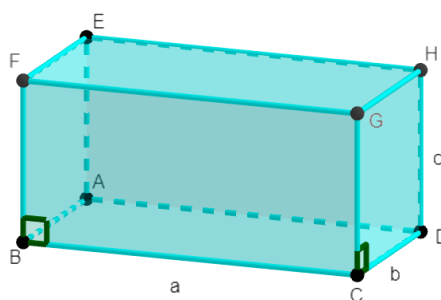
Figura 44 - Paralelepípedo Retângulo
