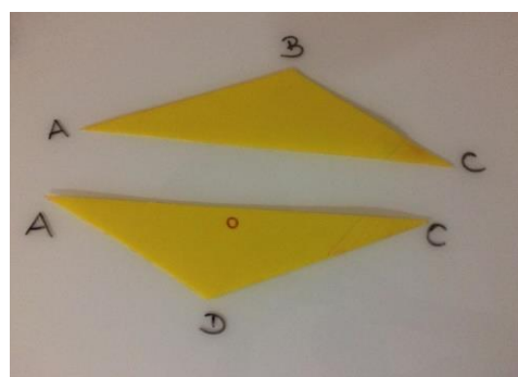
Figura 88 – Figuras congruentes.
