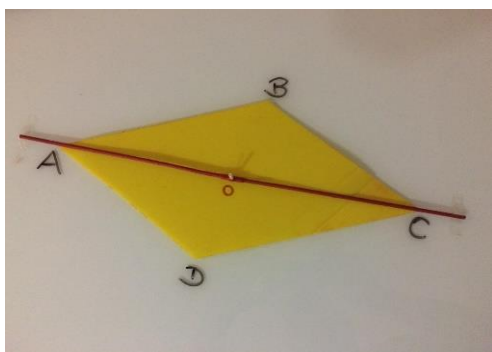
Figura 87 – Primeiro paralelogramo.
