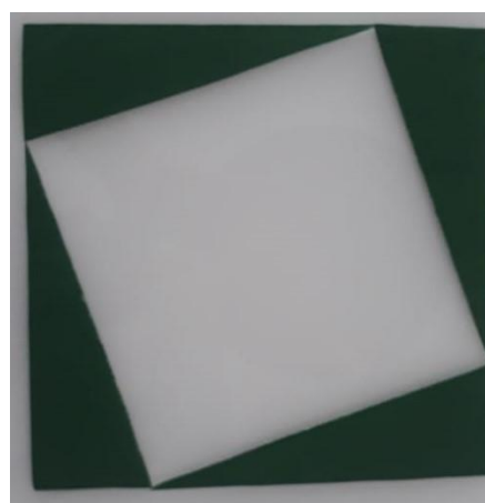
Figura 150 – 2ª composição.
