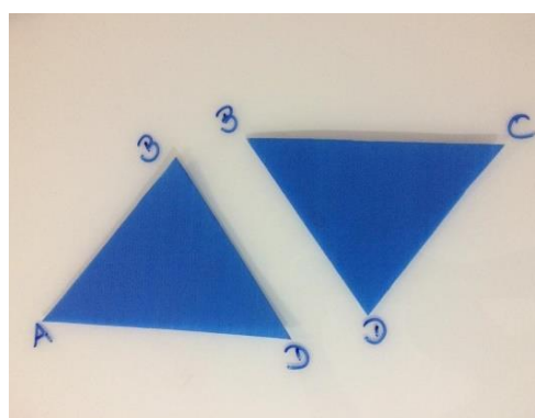
Figura 92 – Formas congruentes.
