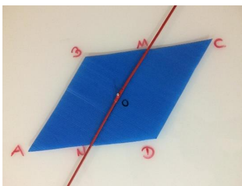
Figura 89 – Segundo paralelogramo.
