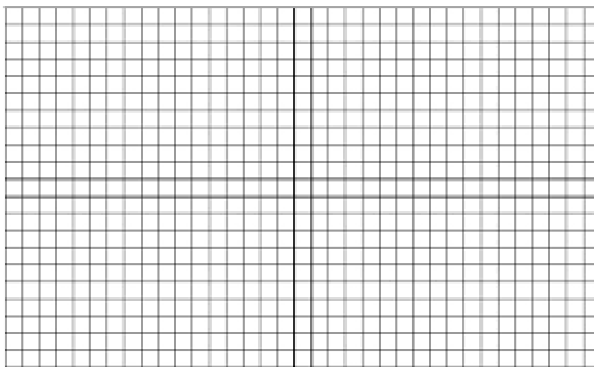
Figura 171 – Malha quadriculada.
