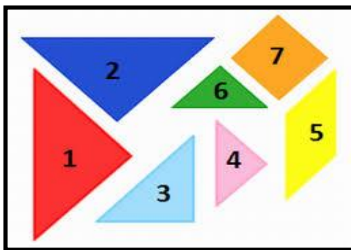
Figura 33 – Peças do Tangram.
