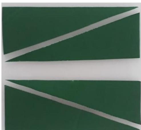
Figura 149 – Triângulos congruentes verdes.
