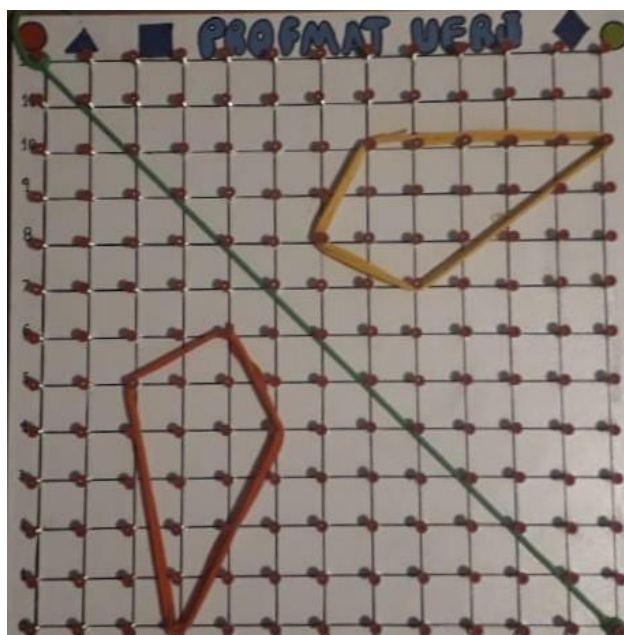
Figura 139 – Imagem da 2ª figura refletida.
