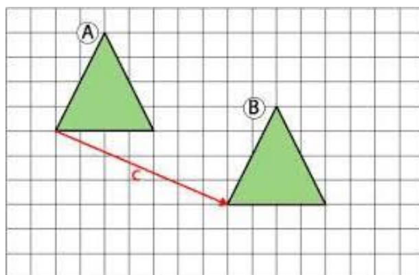
Figura 19 – Translação com um triângulo.
