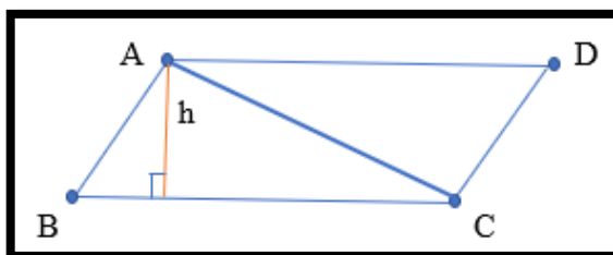
Figura 7 – Paralelogramo ABCD.
