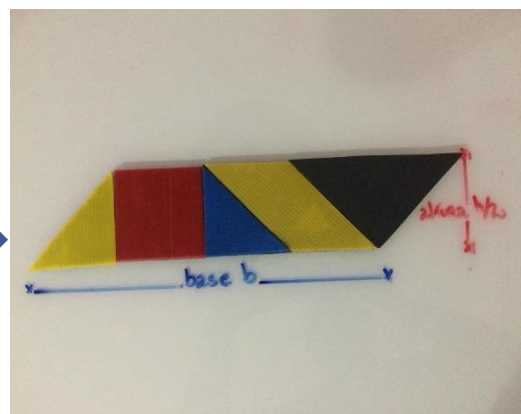
Figura 40 – Paralelogramo formado.
