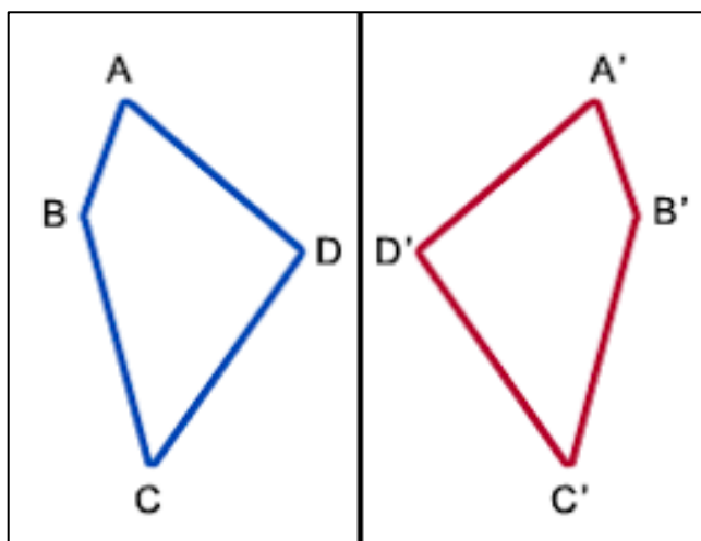
Figura 20 – Reflexão do quadrilátero ABCD.
