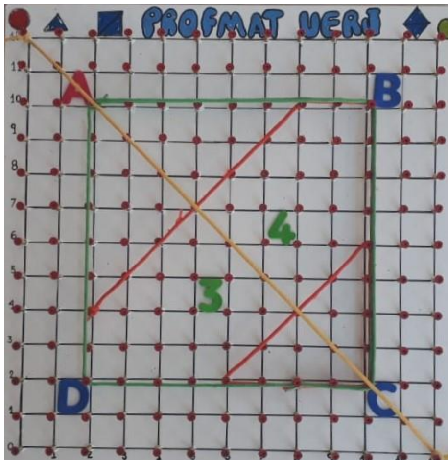
Figura 188 – 2ª representação da atividade 4.
