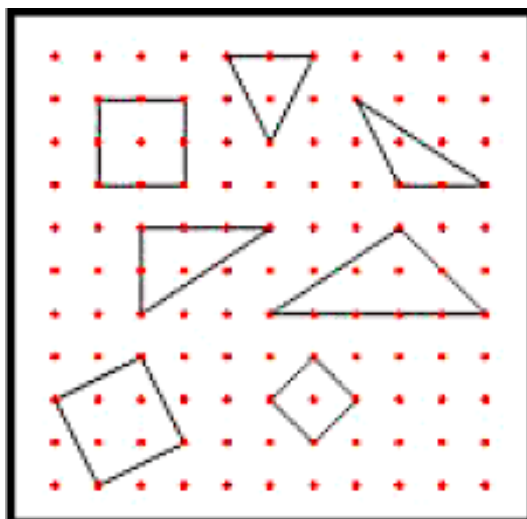
Figura 132 – Geoplano quadriculado.
