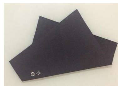
Figura 121 – Dobradura “C”.
