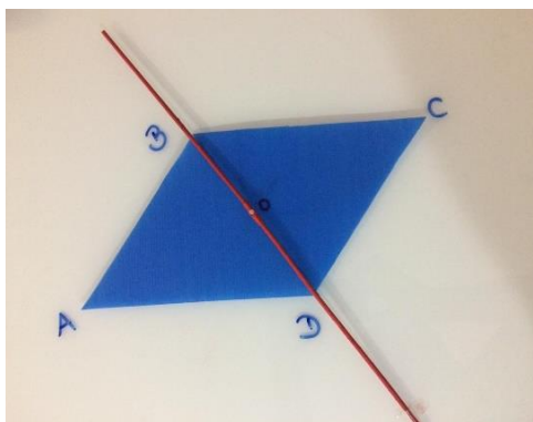
Figura 91 – Terceiro paralelogramo.
