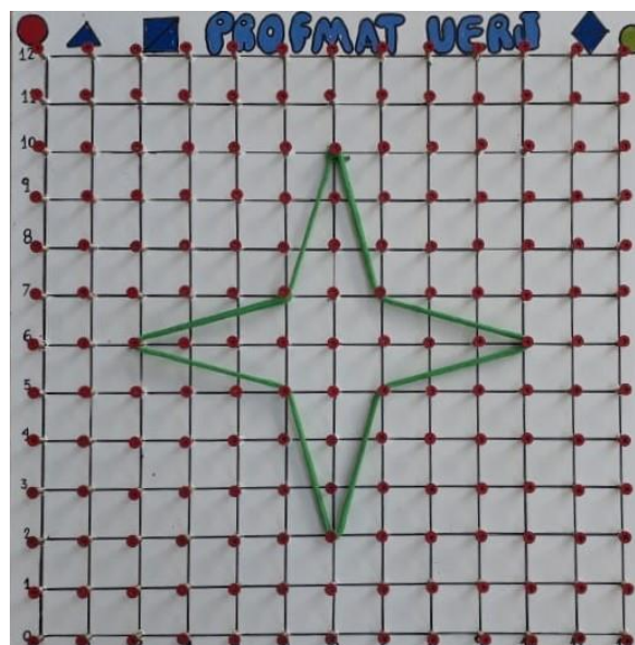
Figura: 162 – Estrela de 4 pontas no Geoplano.
