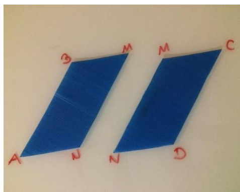
Figura 90 – Polígonos congruentes.
