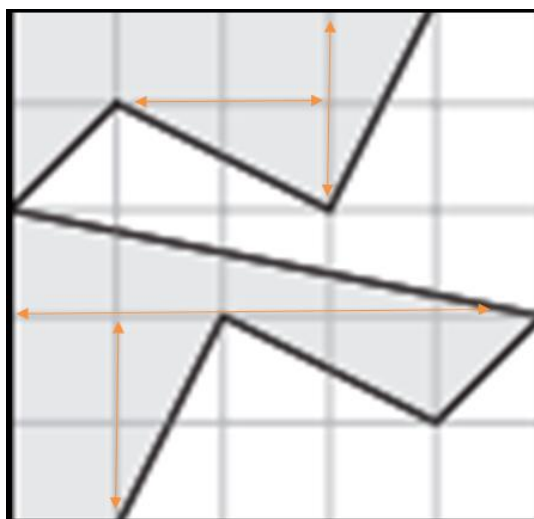
Figura 177 – Área desejada decomposta.
