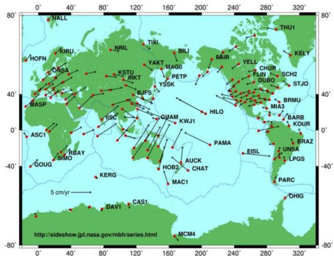
FIGURA 7. MOVIMENTOS DAS PLACAS TECTÔNICAS
