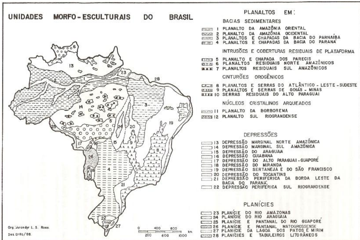
Figura 6. A classificação de Ross sobre o relevo brasileiro
