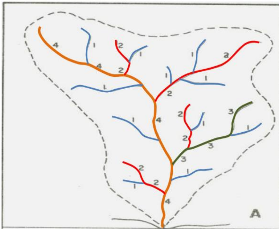
FIGURA 15. REPRESENTAÇÃO DA CLASSIFICAÇÃO DE HORTON
