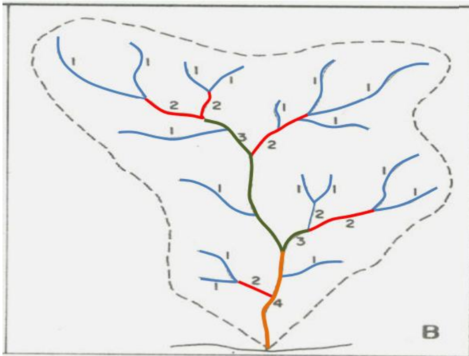
FIGURA 16. REPRESENTAÇÃO DA CLASSIFICAÇÃO DE STRAHLER
