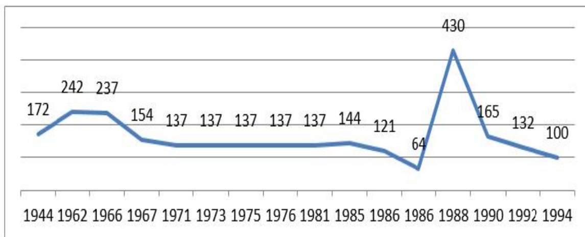
GRÁFICO 1. GRÁFICO DOS ÍNDICES PLUVIOMÉTRICOS
