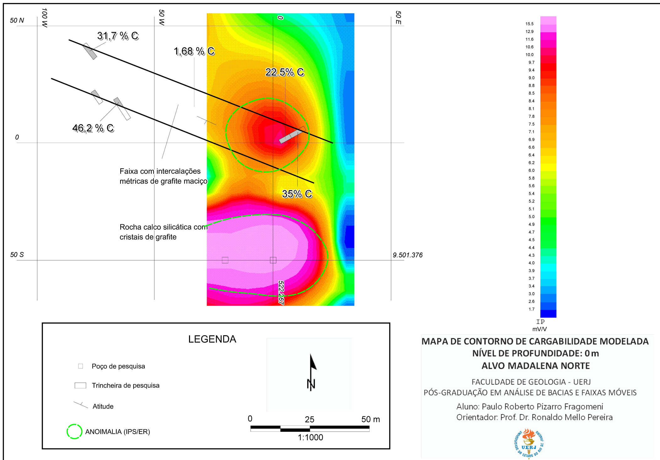
Figura 61 – Mapa geológico do alvo Madalena Norte
