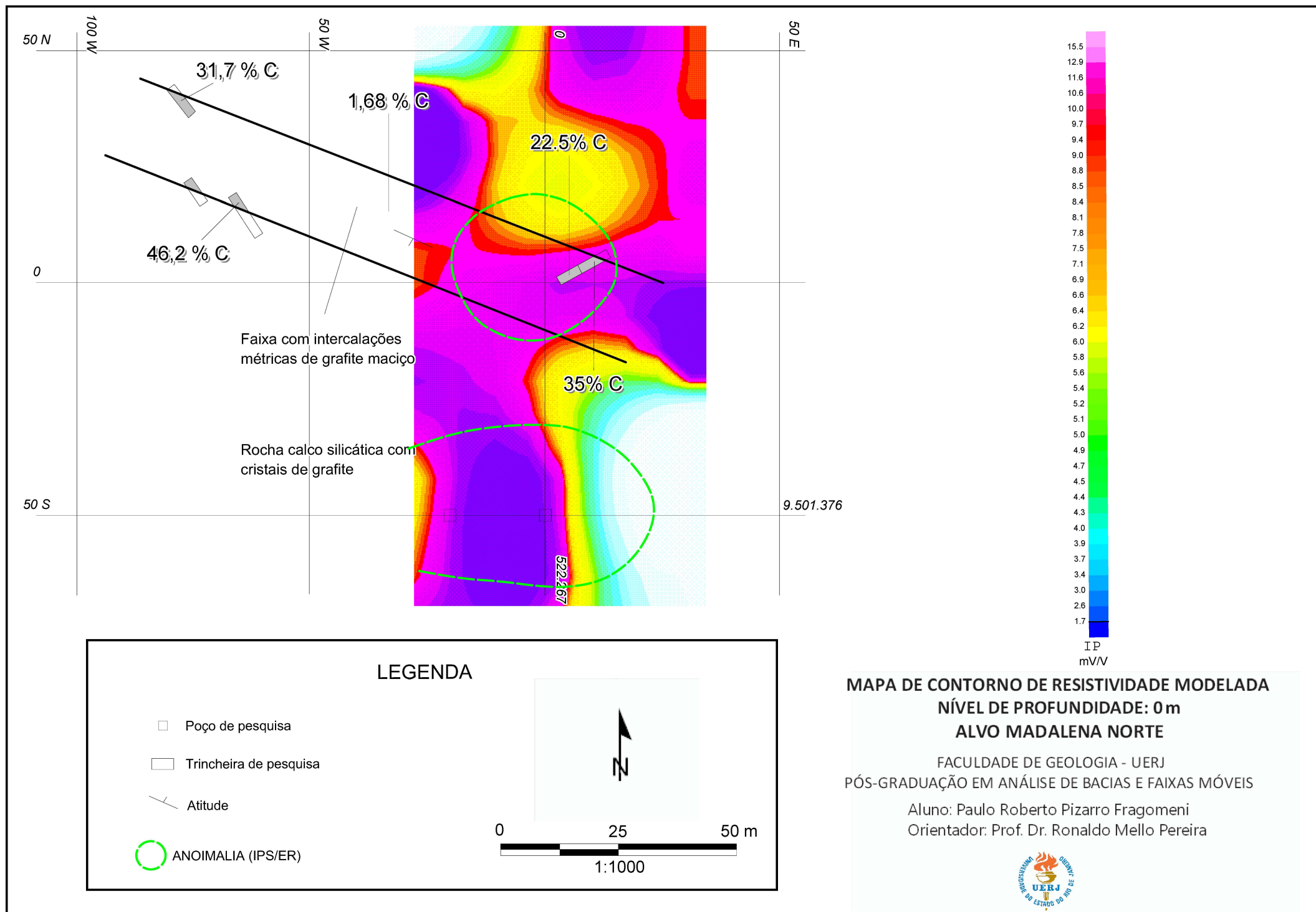
Figura 62 – Mapa de cargabilidade (IPS) do alvo Madalena Norte
