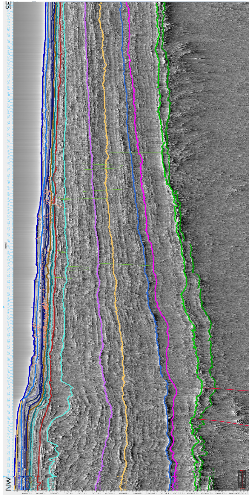
Figura 20. Linha sísmica 1800 (TecVa) e interpretada em profundidade.
