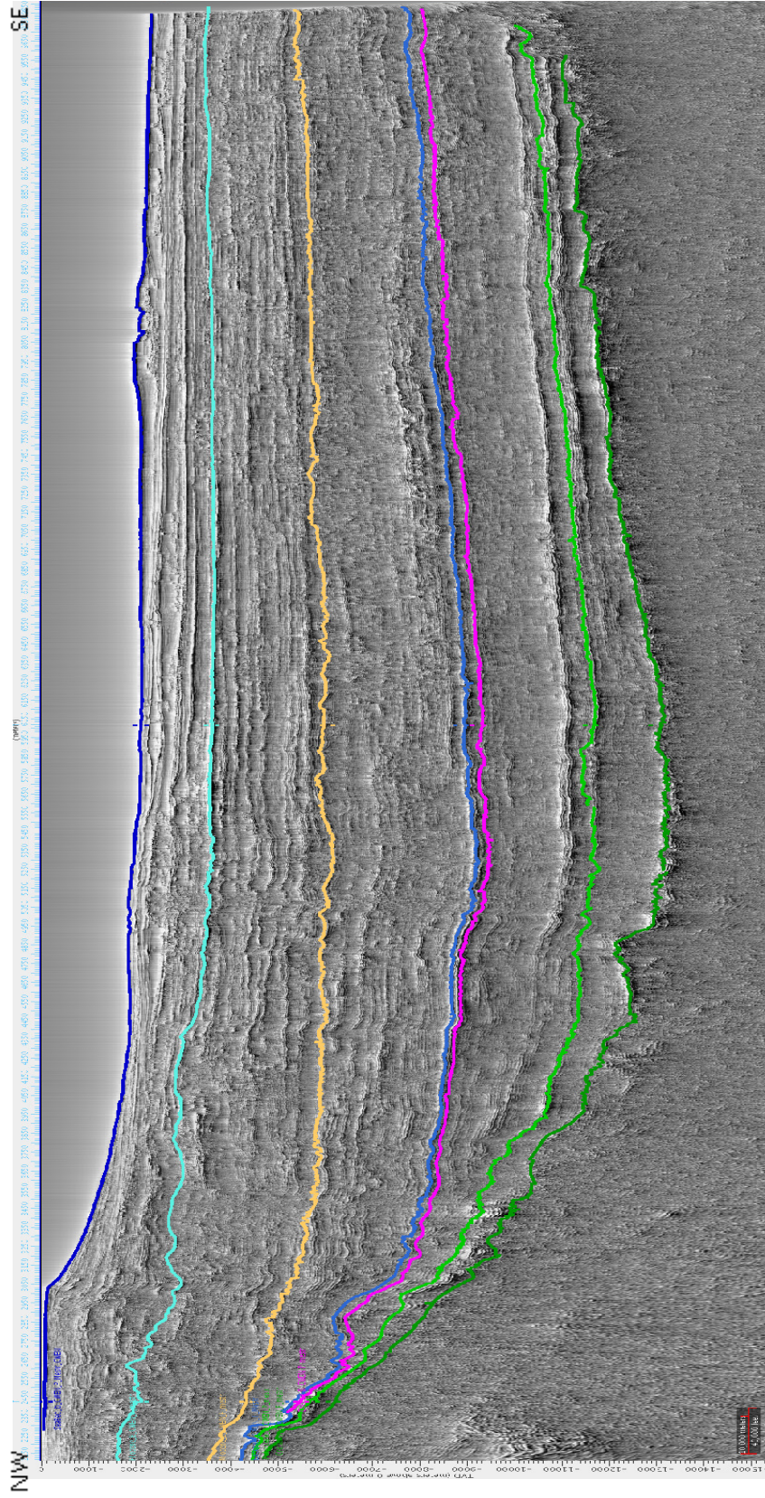
Figura 21. Linha sísmica 1700 (TecVa) e interpretada em profundidade.
