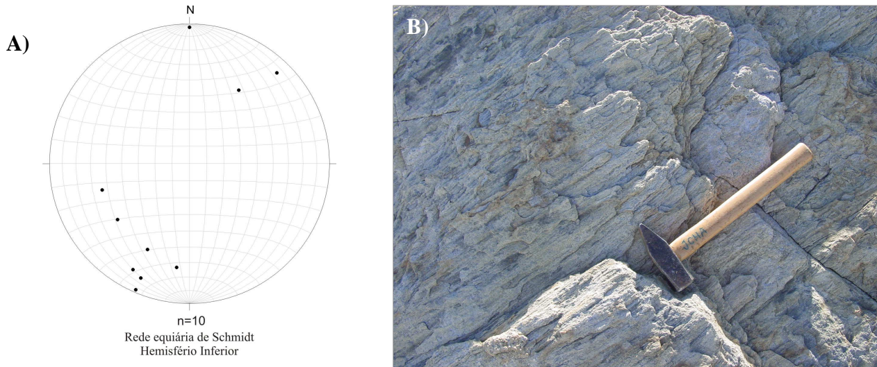
Figura 35 - a) Estereograma de lineações, mostrando predomínio de mergulho para SW com baixo ângulo; b) Forte lineação em rocha granitóide, formado por estiramento de feldspato na Ilha do Mel. Ponto POP-DJL-10.
