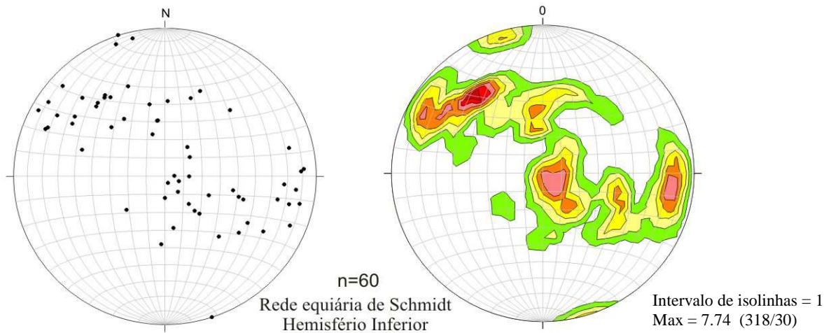
Figura 33 - Estereograma dos pólos da foliação principal S_n , e diagrama de densidade, mostrando direção de foliação NE-SW, com ângulos de mergulho variados, com máxima ocorrência mergulhando para SE, com ângulo médio a alto . Isolinhas = 1.
