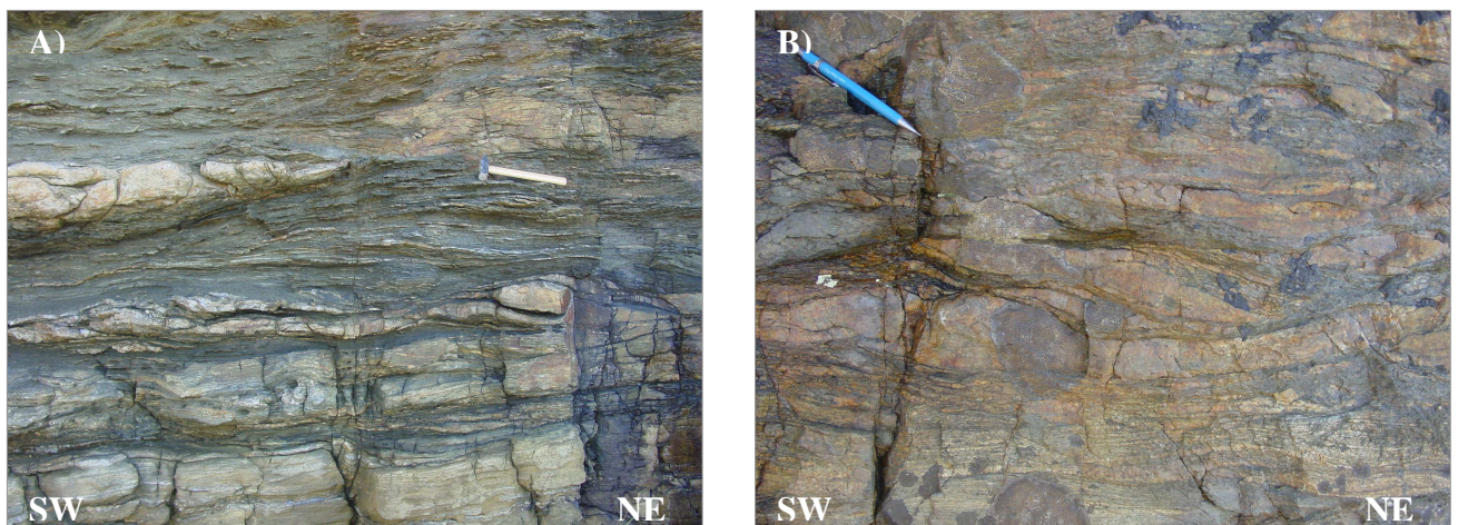
Figura 34: a) Migmatito bandado, com porção máfica mais micácea, apresentando xistosidade e porção clara de fusão quartzo-feldspática.; b) Sigmóide formado na porção fundida, Gruta das Encantadas – Ilha do Mel . Ponto POP-DJL-07.
