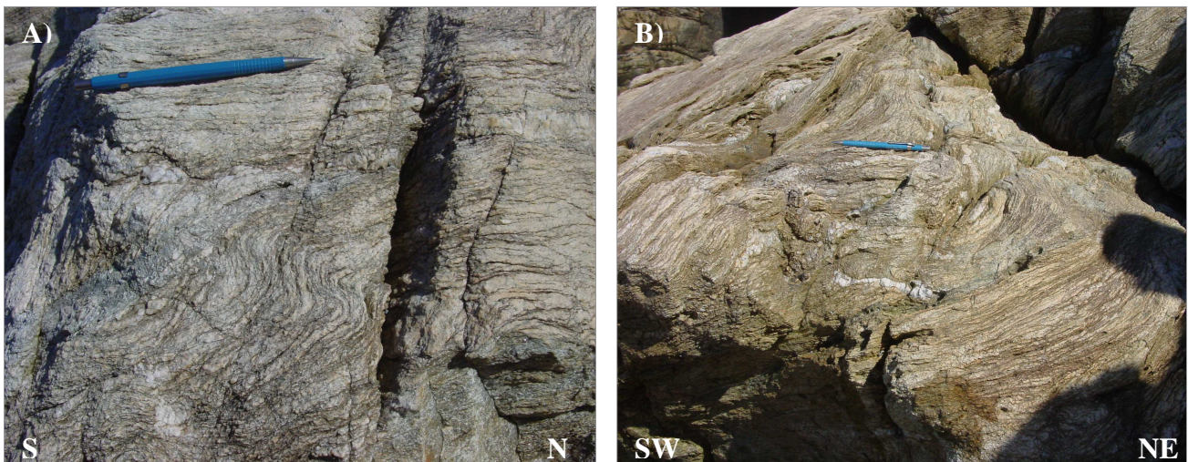
Figura 36 - A) Dobras em S nas rochas do Complexo São Francisco do Sul; B) Dobras suaves irregulares, Gruta das Encantadas – Ilha do Mel. POP-DJL-07.
