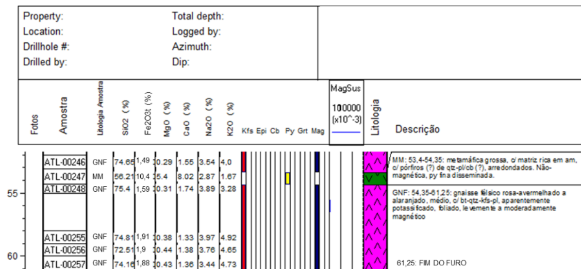
Figura 56 - Log geológico do furo CG-SB-DDH-0002 (continuação)
