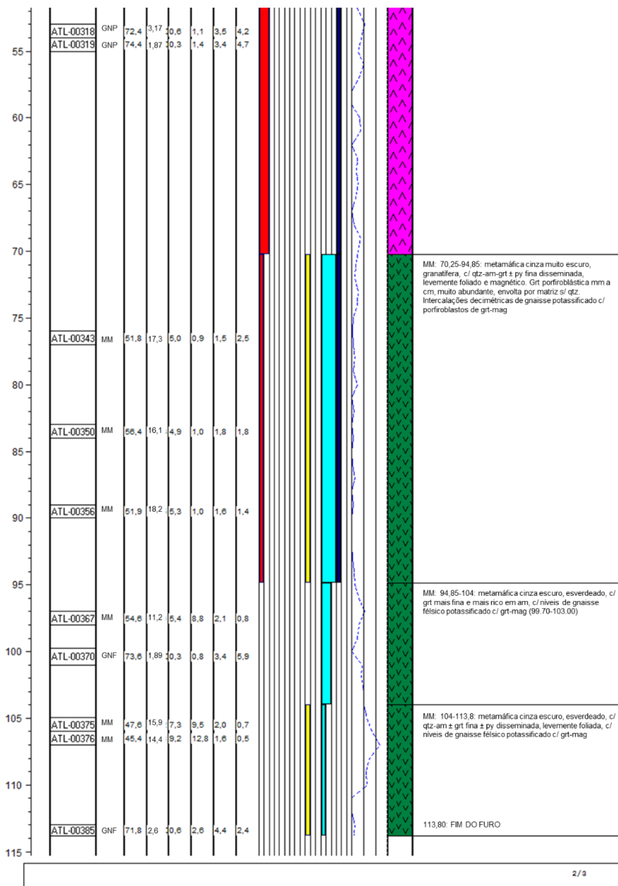
Figura 57 - Log geológico do furo CG-SB-DDH-0003 (continuação)
