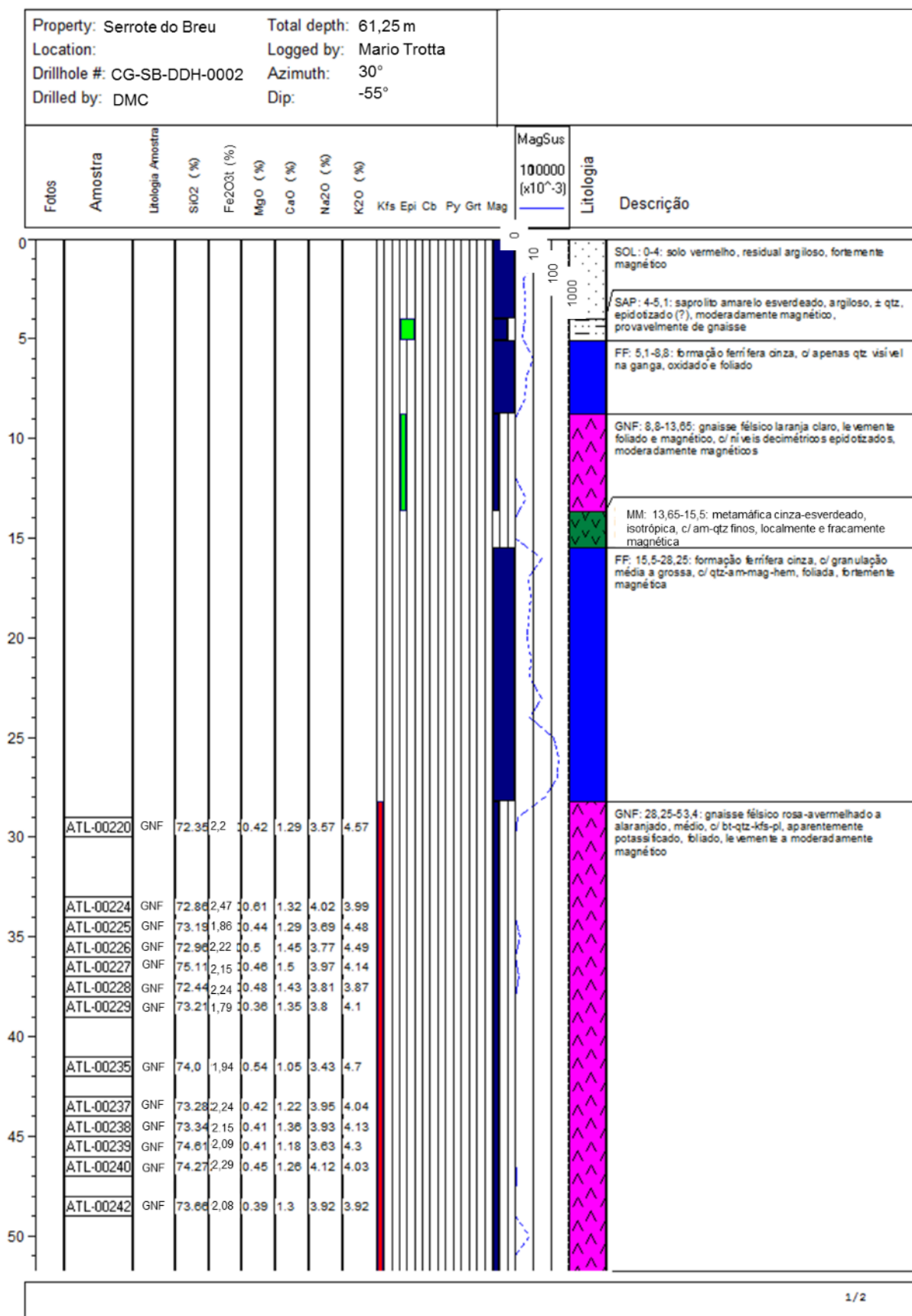
Figura 56 - Log geológico do furo CG-SB-DDH-0002 (continua)
