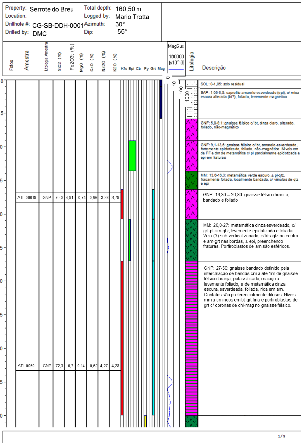
Figura 55 – Log geológico do furo CG-SB-DDH-0001 (continua)
