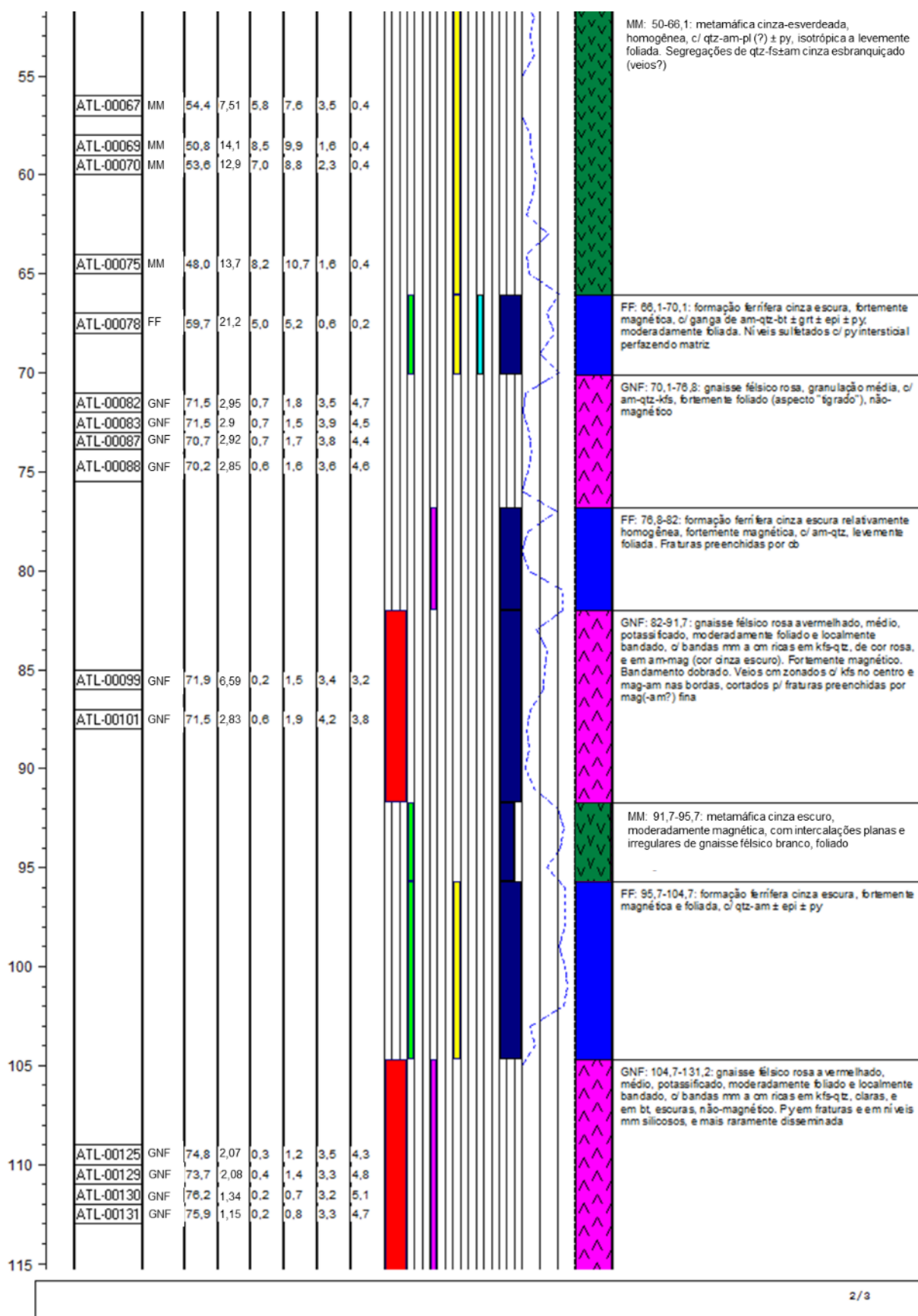
Figura 55 – Log geológico do furo CG-SB-DDH-0001 (continuação)
