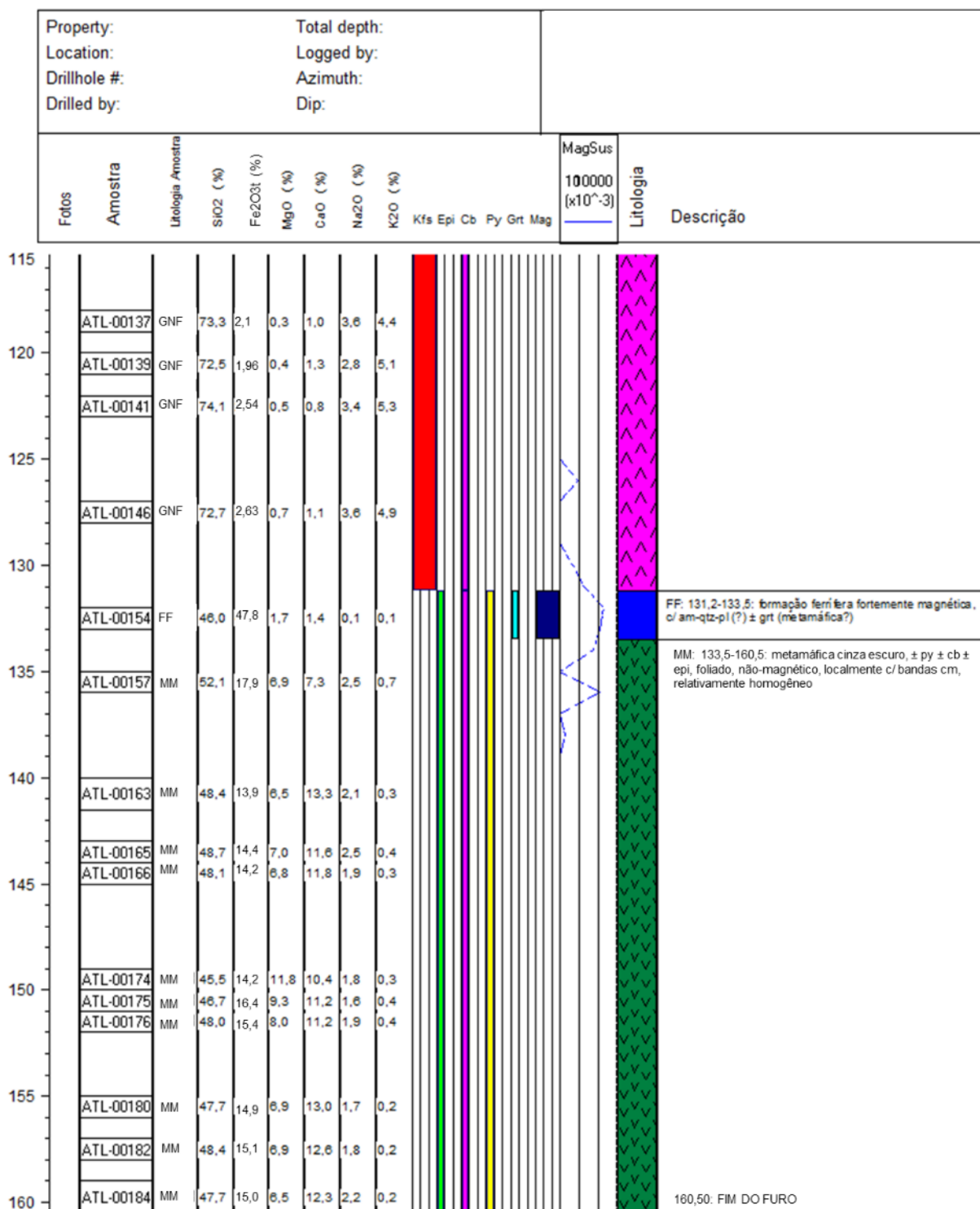
Figura 55 – Log geológico do furo CG-SB-DDH-0001 (continuação)
