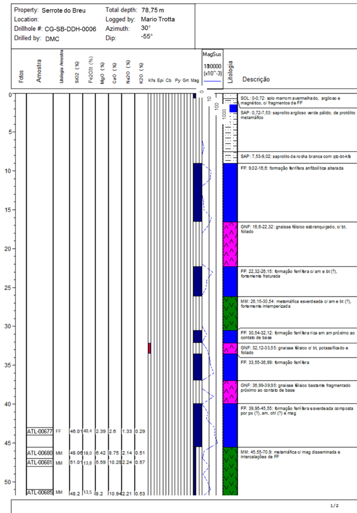
Figura 60 - Log geológico do furo CG-SB-DDH-0006 (continua)
