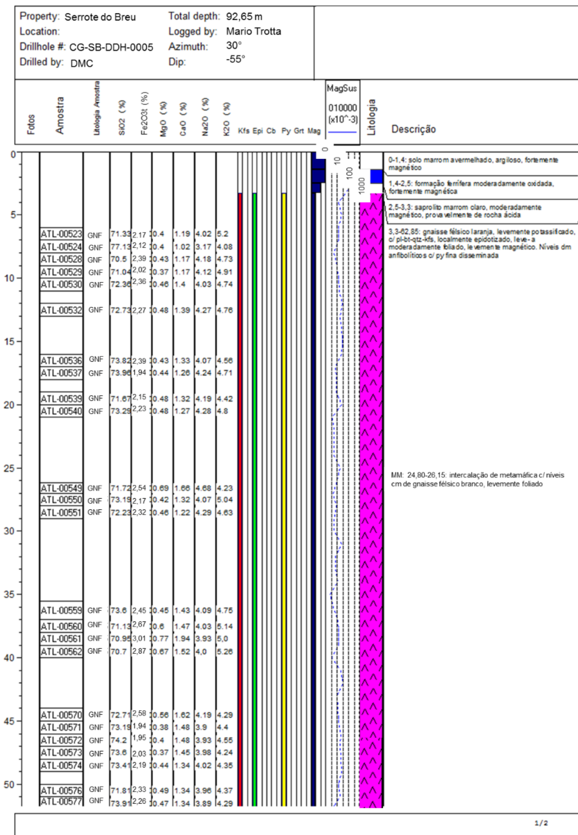
Figura 59 - Log geológico do furo CG-SB-DDH-0005 (continua)
