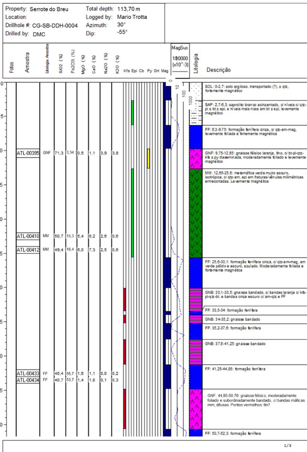
Figura 58 - Log geológico do furo CG-SB-DDH-0004 (continua)
