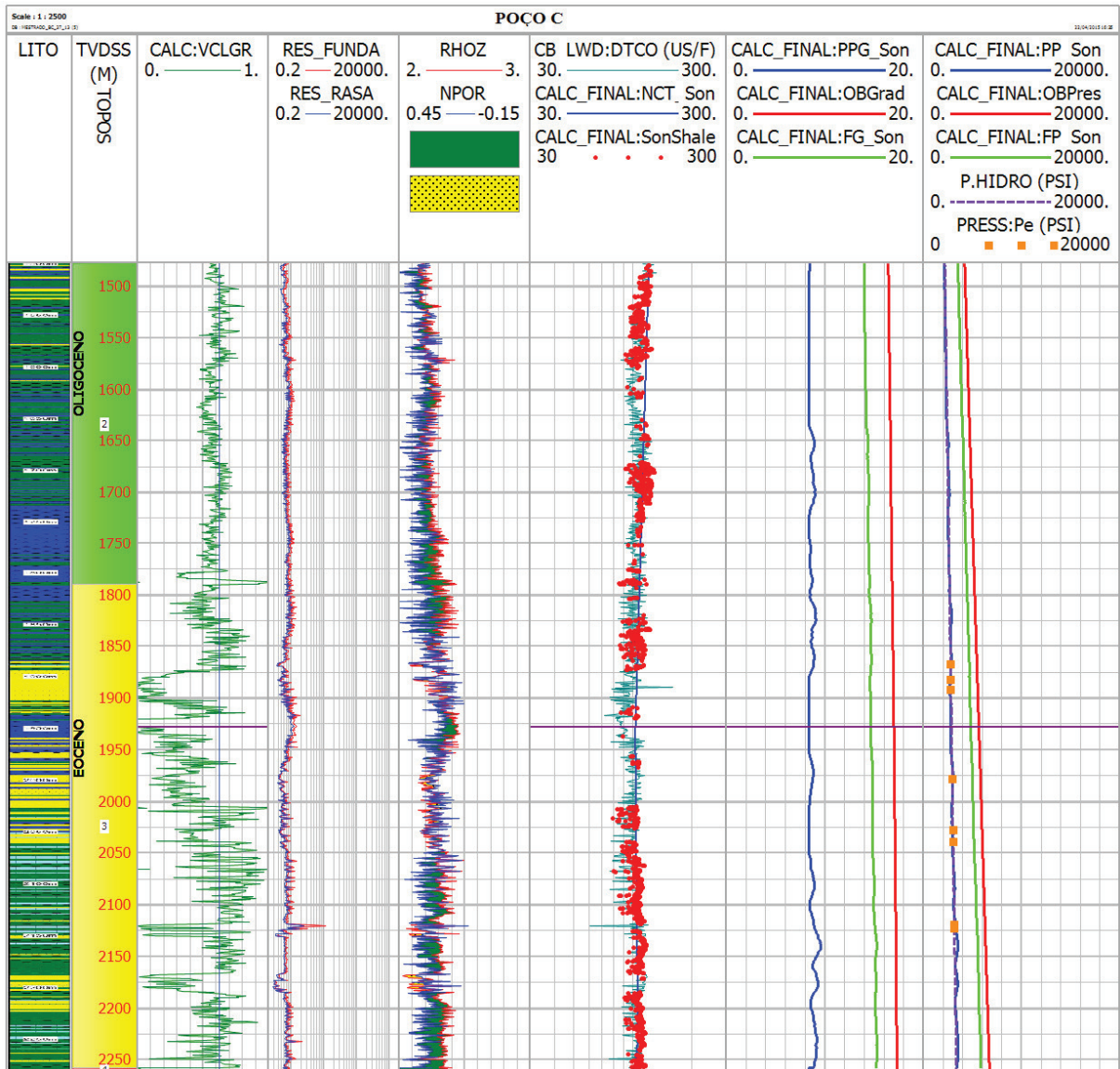
Figura 30 - Perfil resultante de cálculo de Pressão de poros normal, intervalo Oligoceno e Eoceno no Poço C
