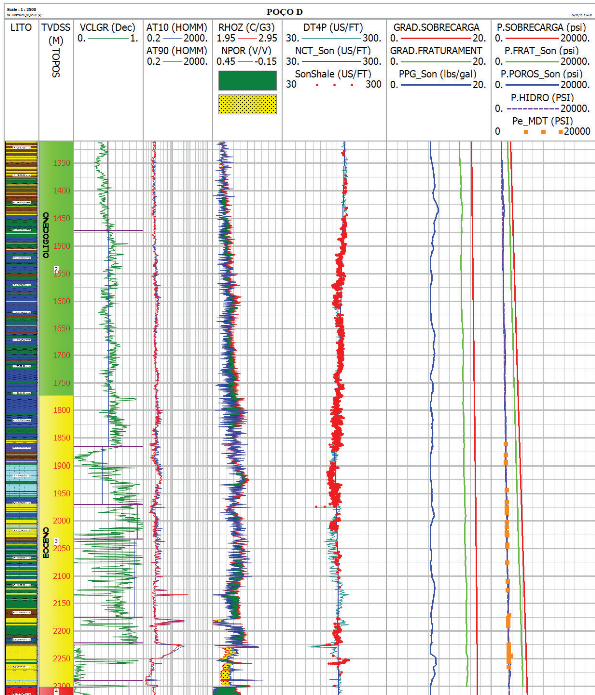
Figura 31 - Perfil resultante de cálculo de Pressão de poros normal, intervalo Oligoceno e Eoceno no poço D
