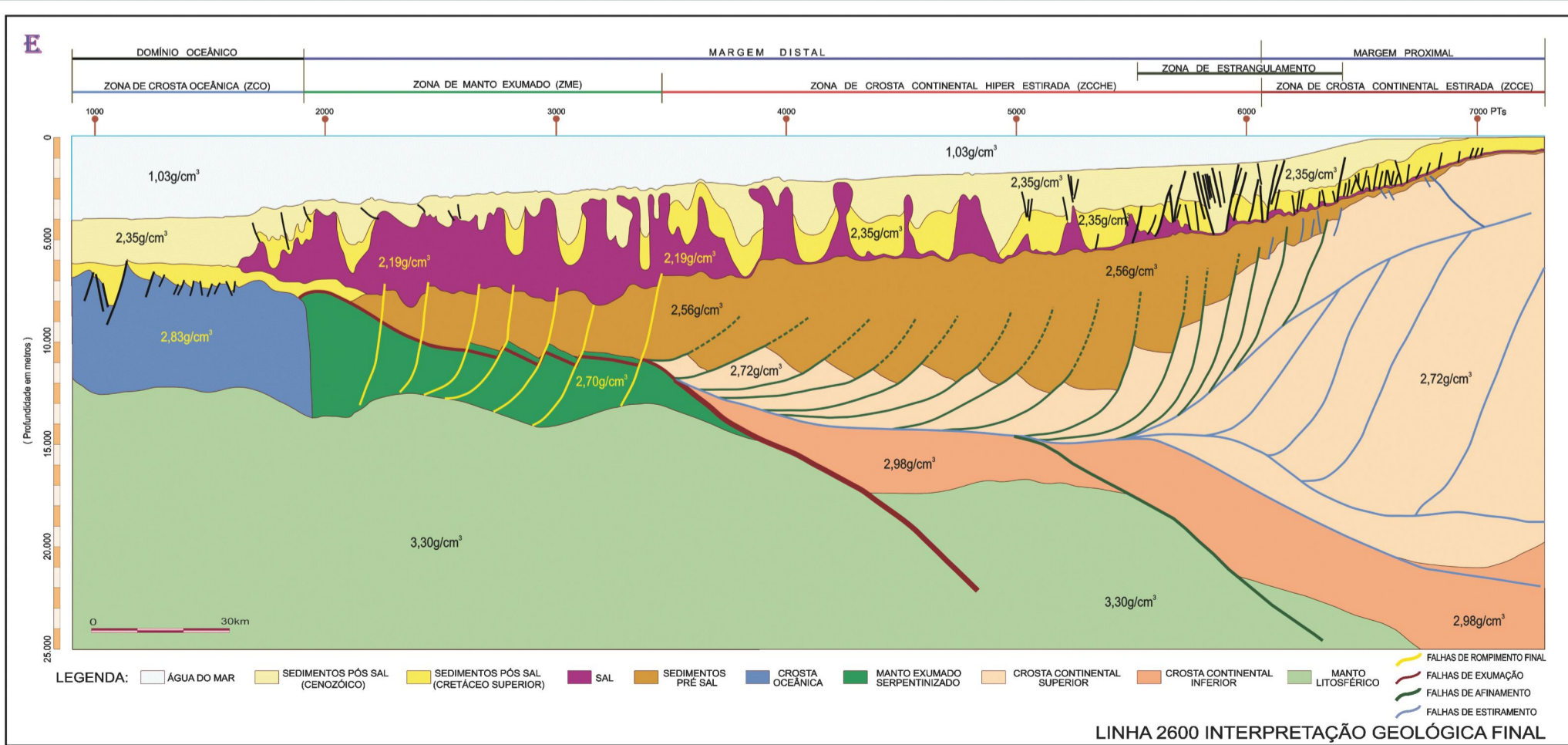
LINHA 2600 ANOMALIA GRAVIMÉTRICA MEDIDA E MODELADA
