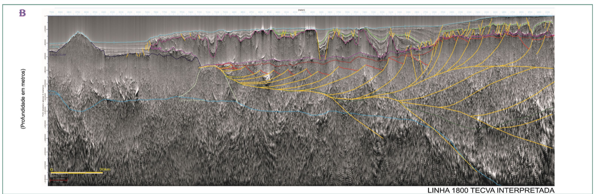
LINHA 1800 TECVA INTERPRETADA
