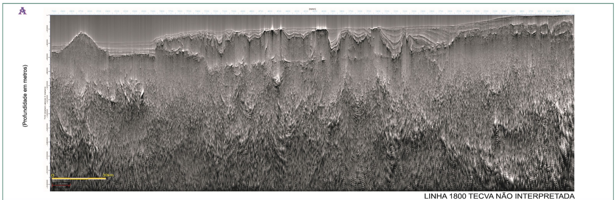
LINHA 1800 TECVA NÃO INTERPRETADA
