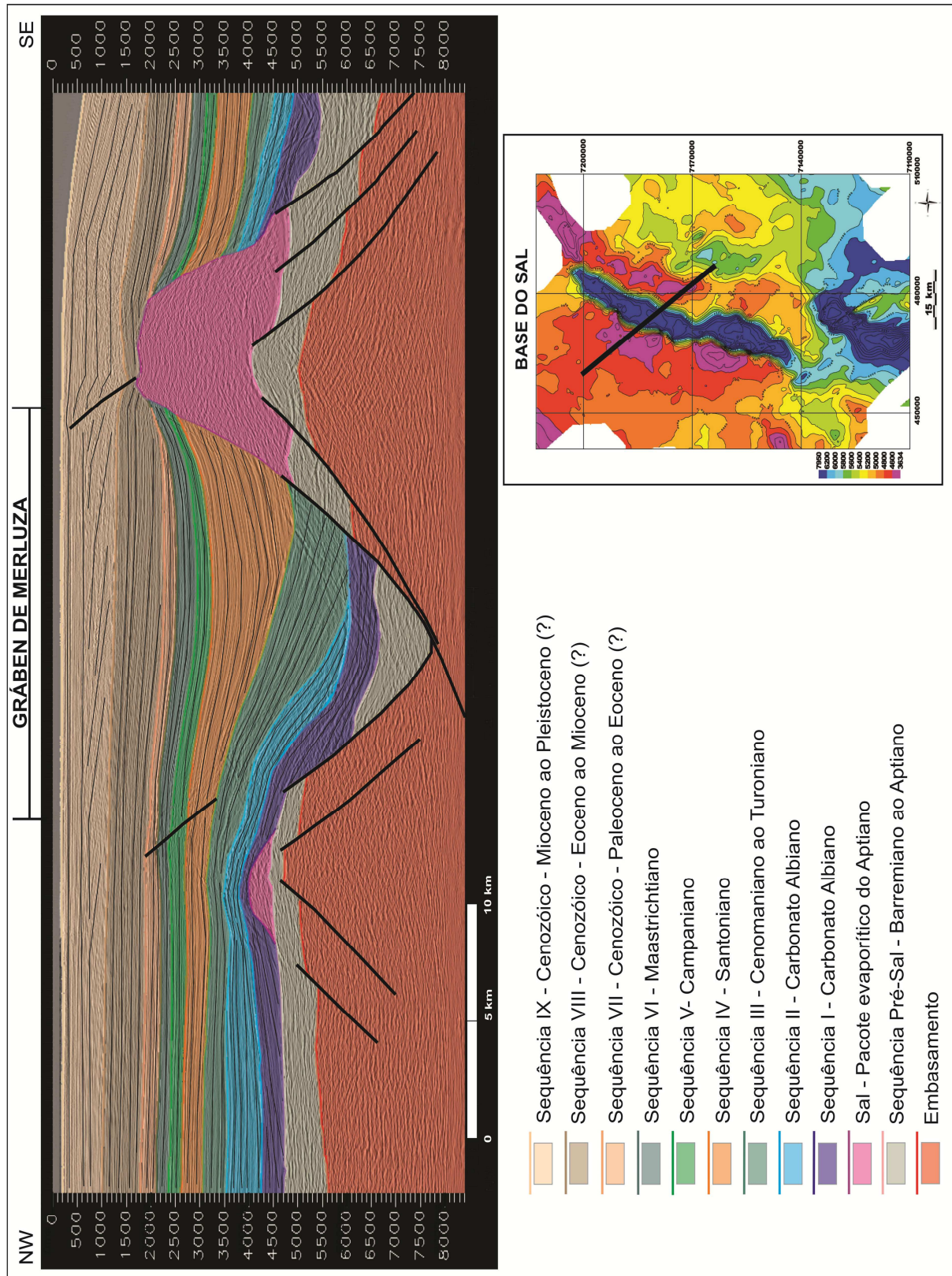
Figura 28: Seção geológica da linha 248-0041.
