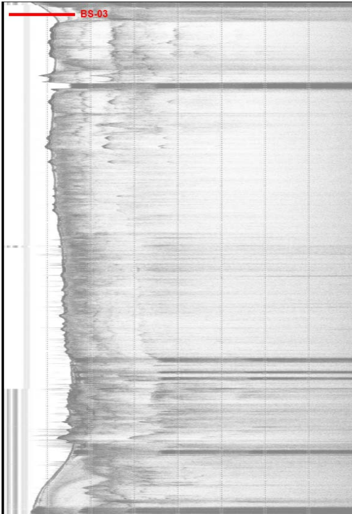
Figura 12 – Perfil Sísmico L2 com a localização do testemunho BS-03 (Villena, 2005).
