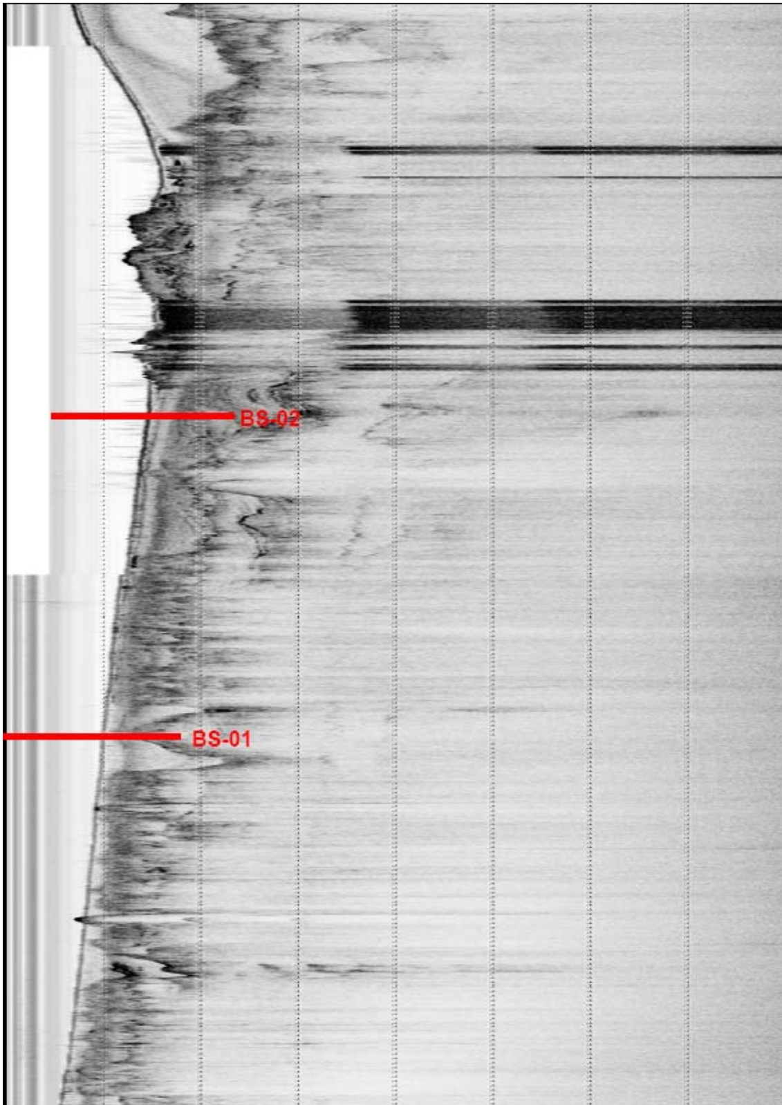
Figura 14 – Perfil Sísmico L4 com a localização dos testemunhos BS-01 e BS-02 (Villena, 2005).
