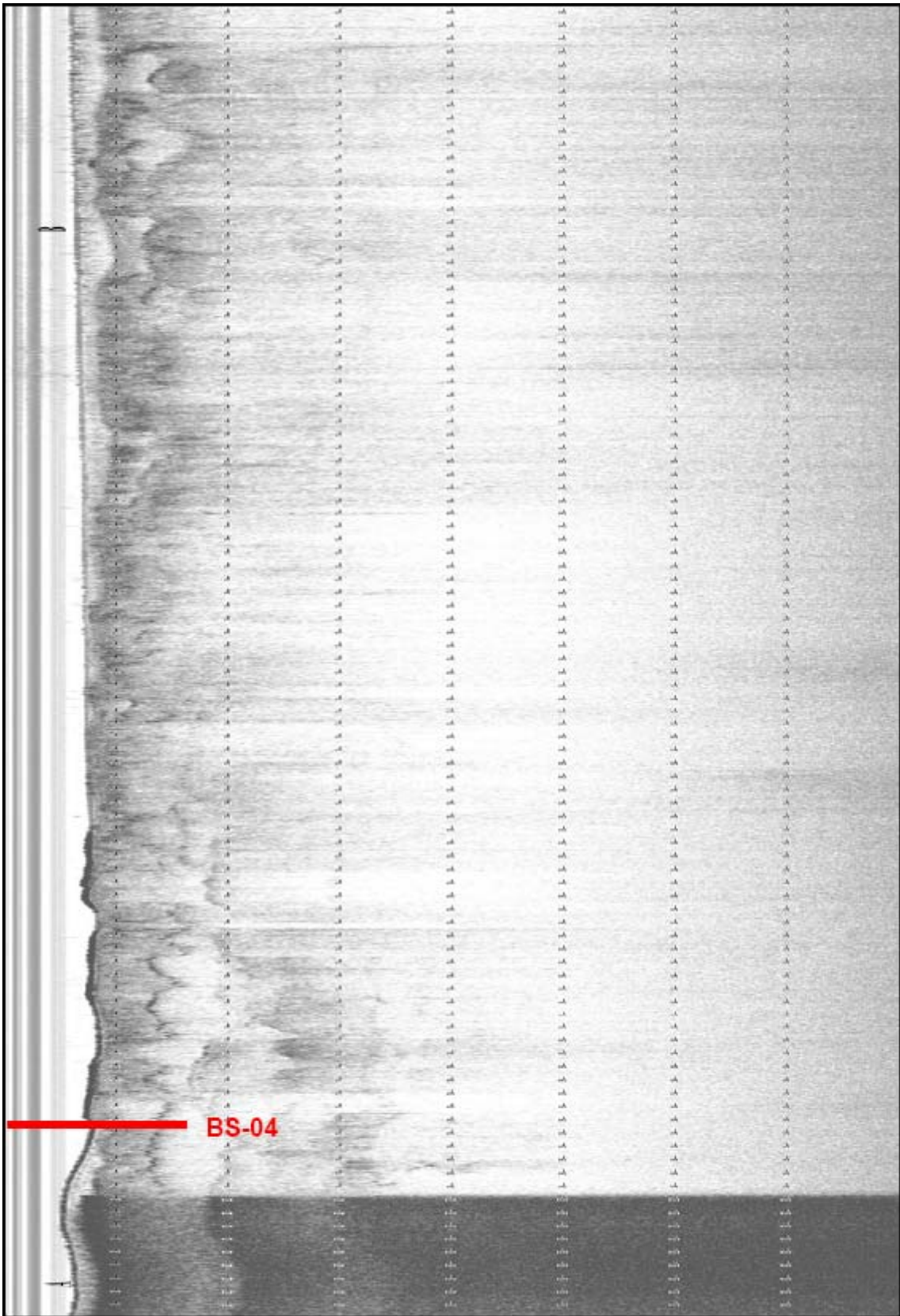
Figura 13 – Perfil Sísmico L3 com a localização do testemunho BS-04 (Villena, 2005).
